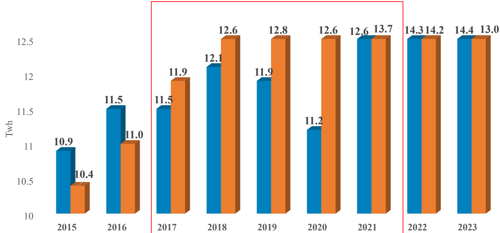
Годичное производство и потребление электроэнергии в Грузии
