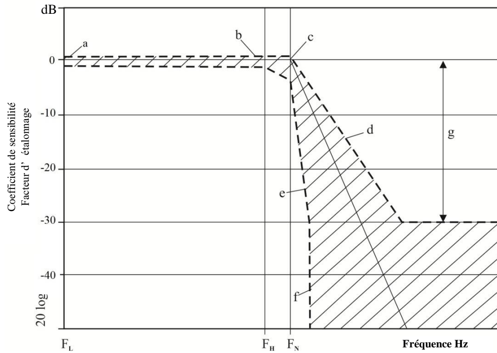
Figure 1 Courbe de réponse en fréquence
