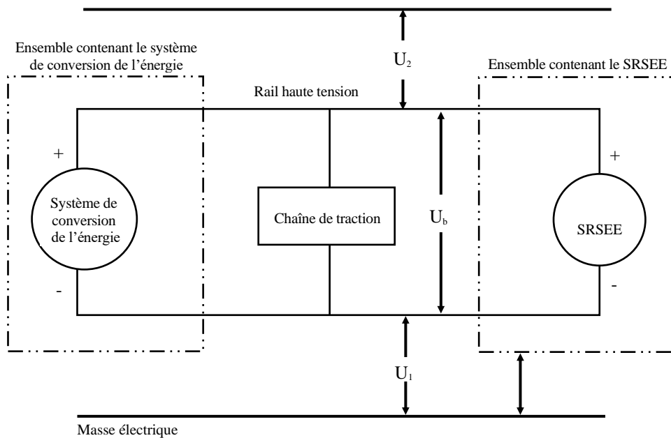
Figure 1 Mesure de U_b , U_1 et U_2
