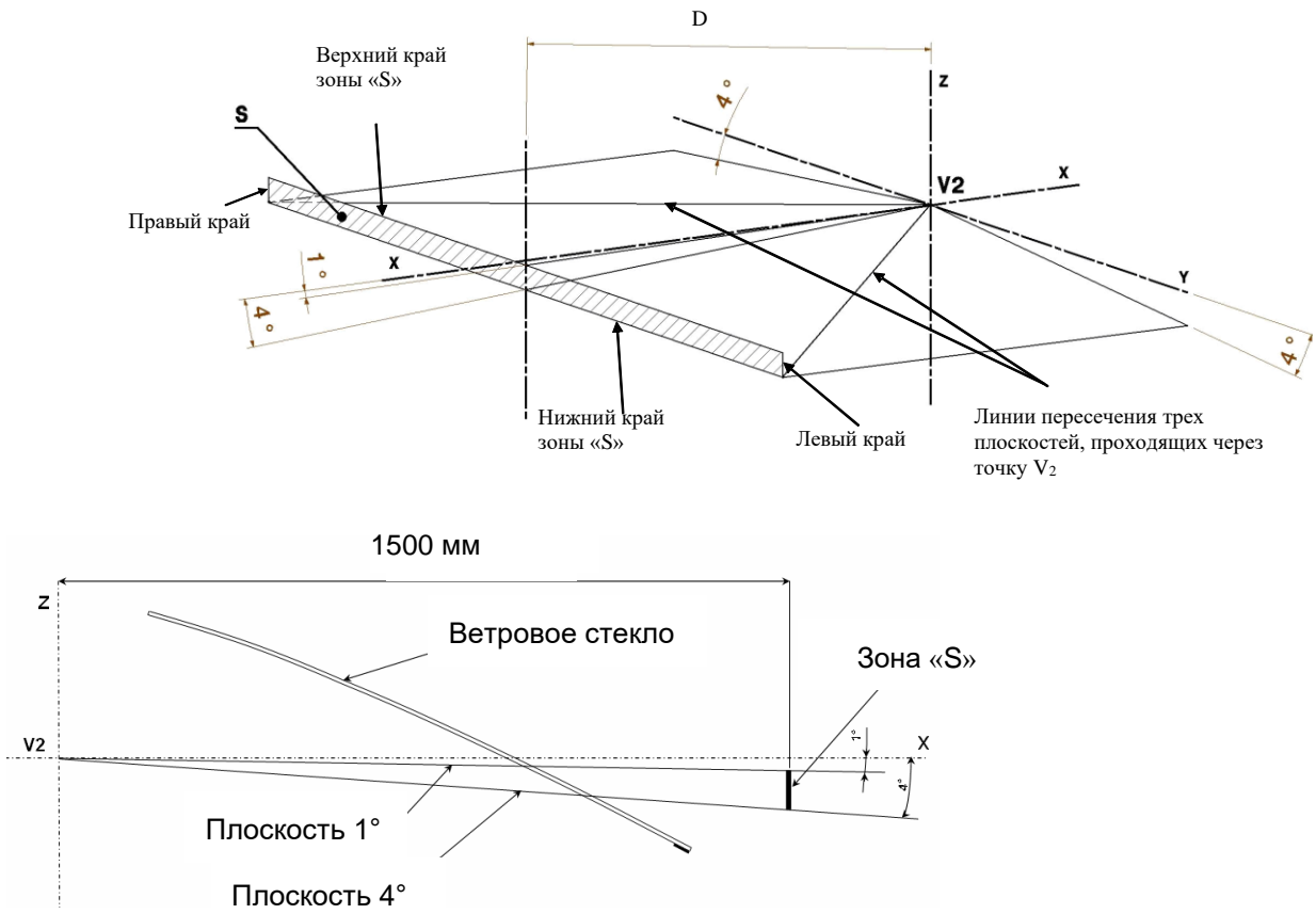
Рис. 7 Определение зоны «S» (см. пункт 5.1.3.2 настоящих Правил)
