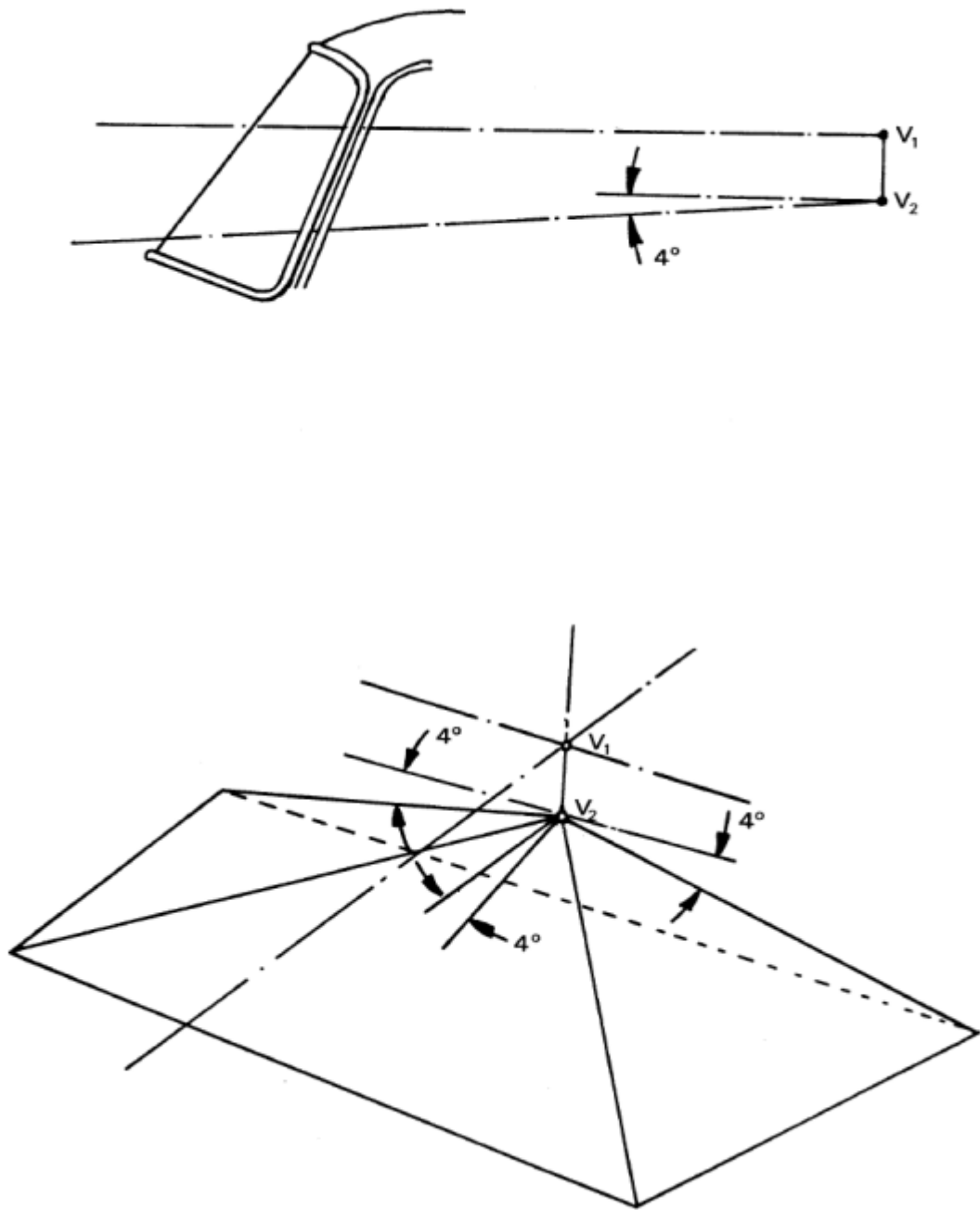
Рис.4 Оценка помех в 180°-м поле обзора водителя спереди
