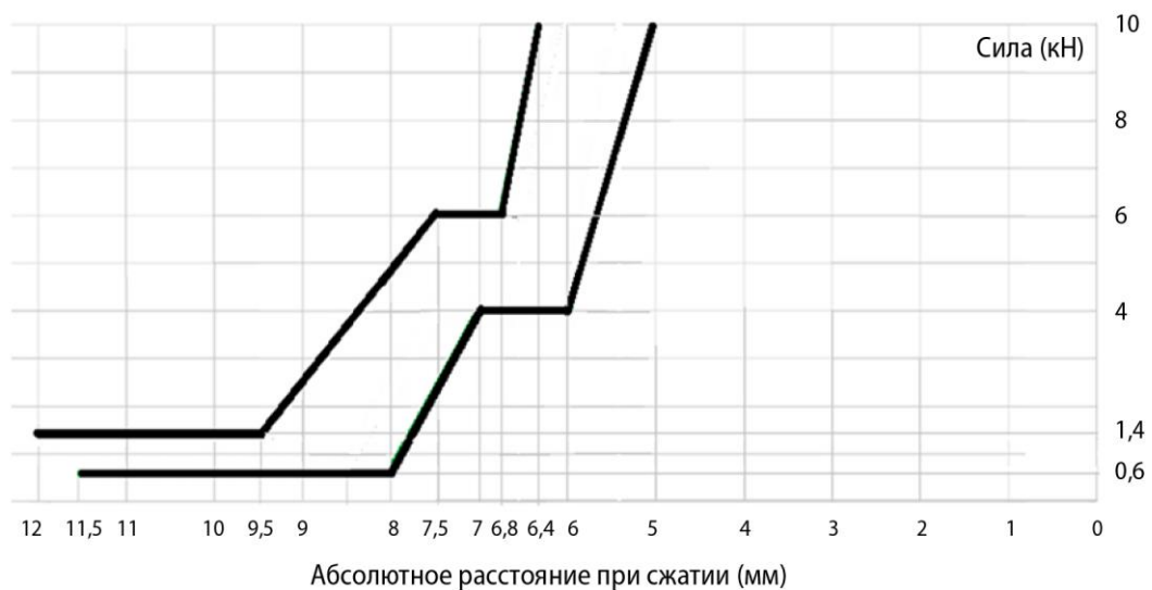
Рис. 6 Коридор на графике соотношения силы и деформации для имитатора динамика
