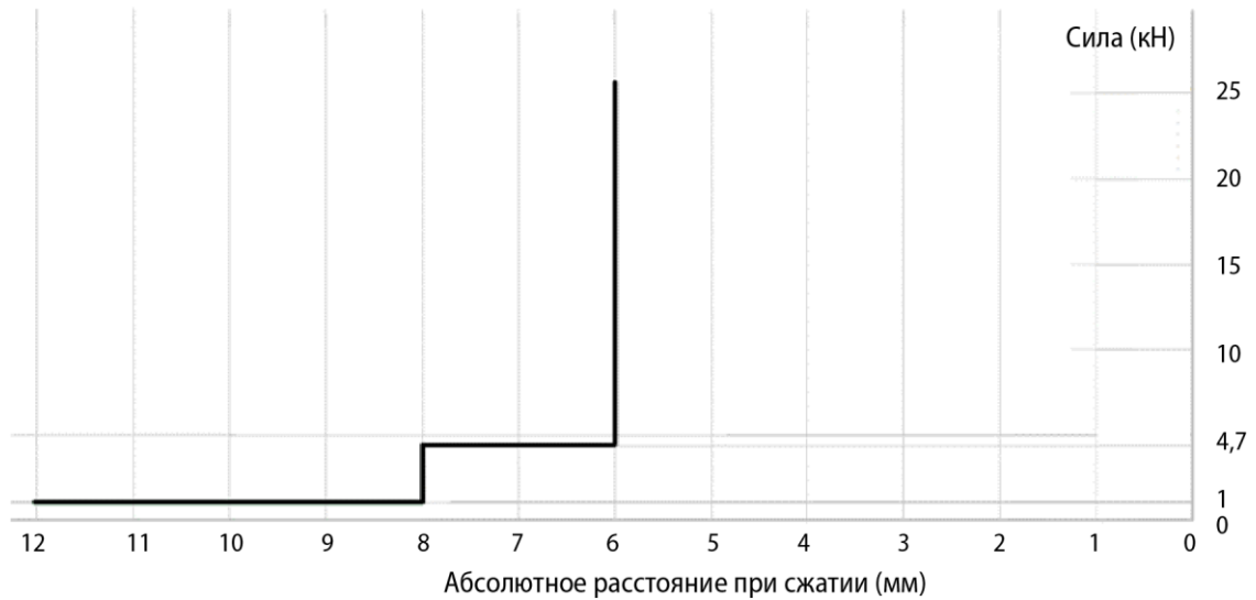
Рис. 4 Коридор для квазистатического испытания на разрушение
