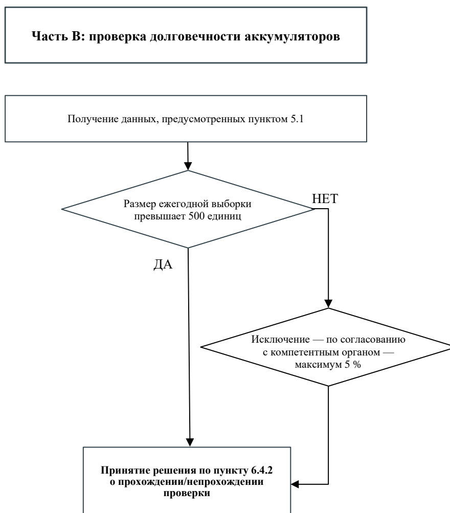
Рис. 2 Блок-схема для части В: проверка долговечности аккумуляторов
