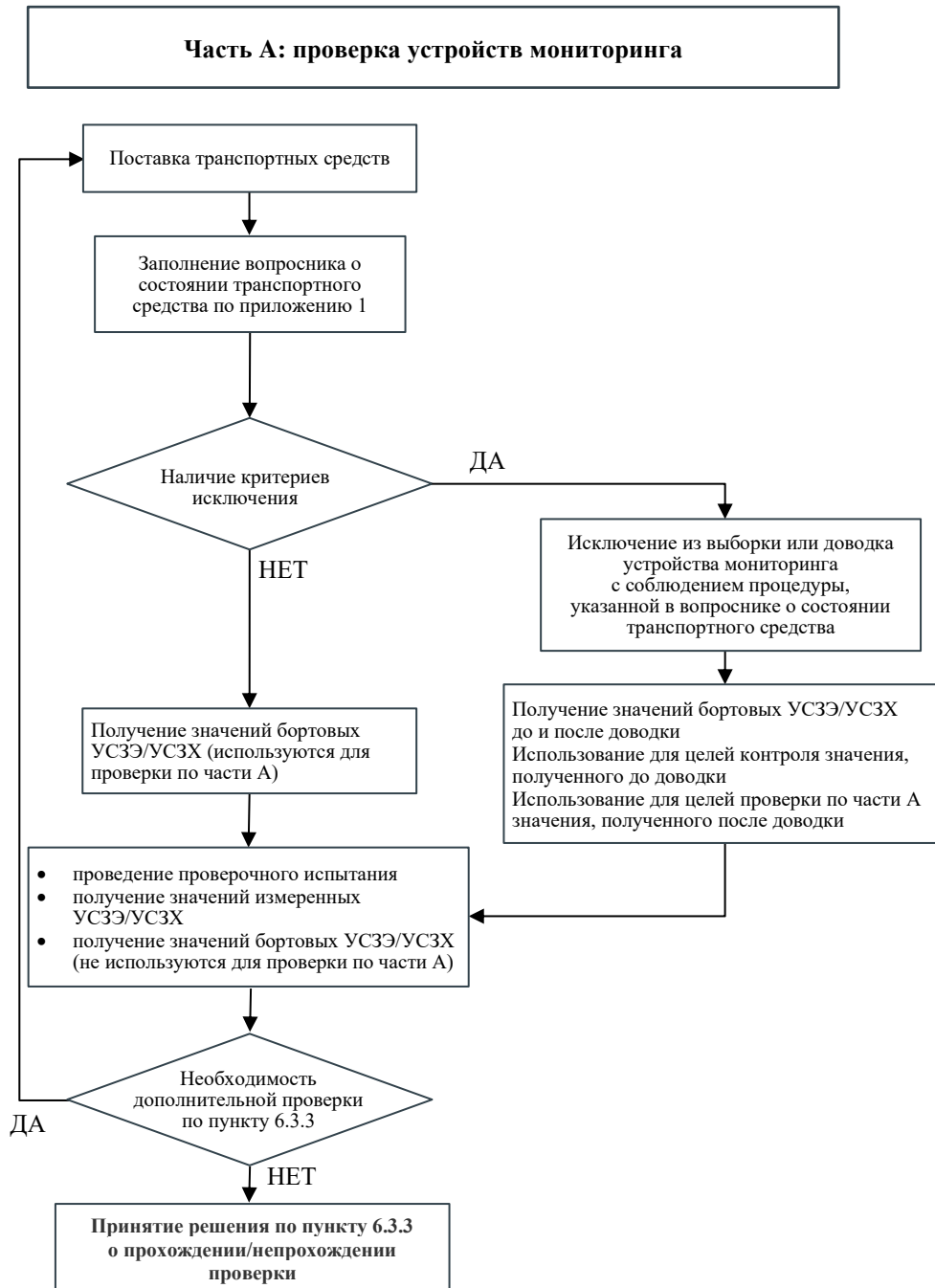
Рис. 1 Блок-схема для части А: проверка устройств мониторинга
