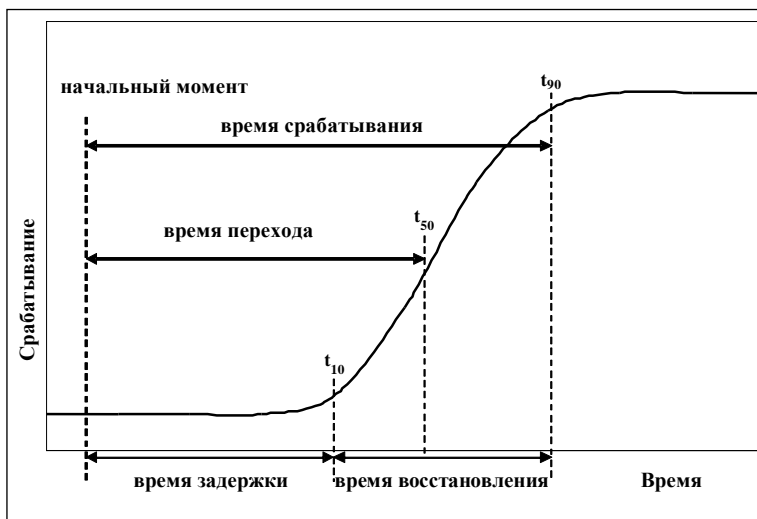
Рис. 1 Определения моментов срабатывания системы
