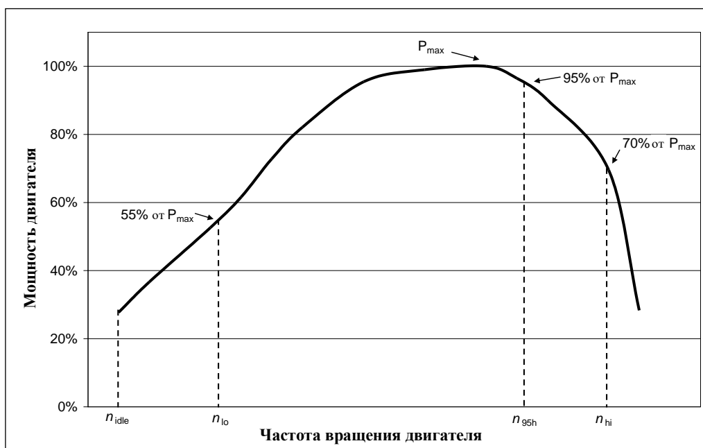
Рис. 4 Определение частот вращения для целей испытаний
