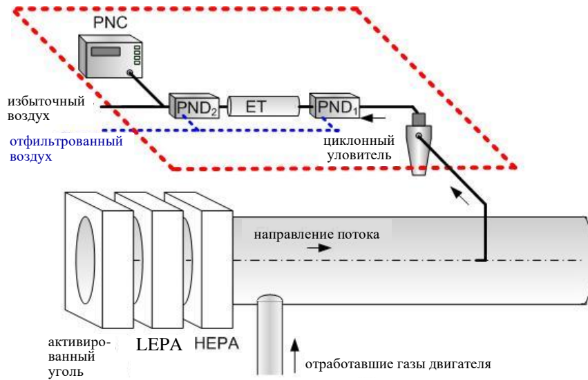
Рис. 20 Принципиальная схема рекомендуемой системы отбора проб частиц: отбор проб с полным разбавлением потока
