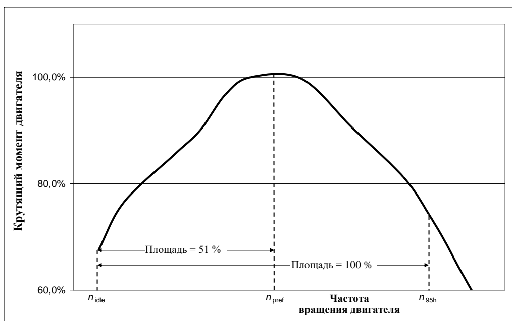
Рис. 5 Определение n_{pref}
