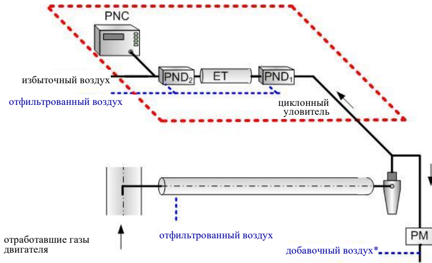
Рис. 19 Принципиальная схема рекомендуемой системы отбора проб частиц: отбор проб с частичным разбавлением потока
