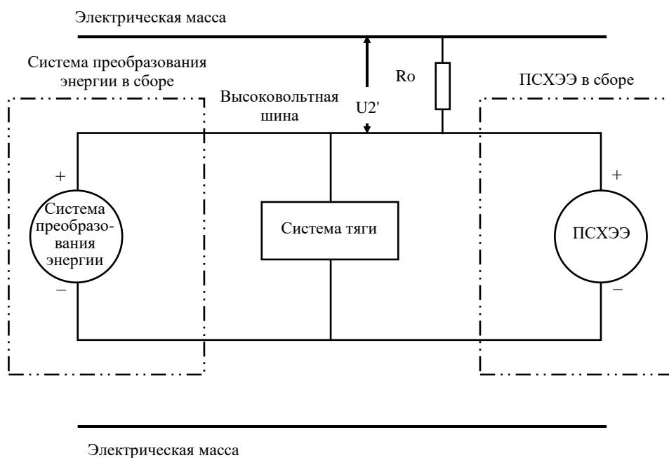
Рис. 6 Измерение U_2'
