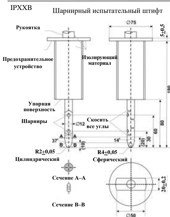
Рис. 3 Шарнирный испытательный штифт Щуп для проверки вероятности прикосновения (Размеры в мм)
