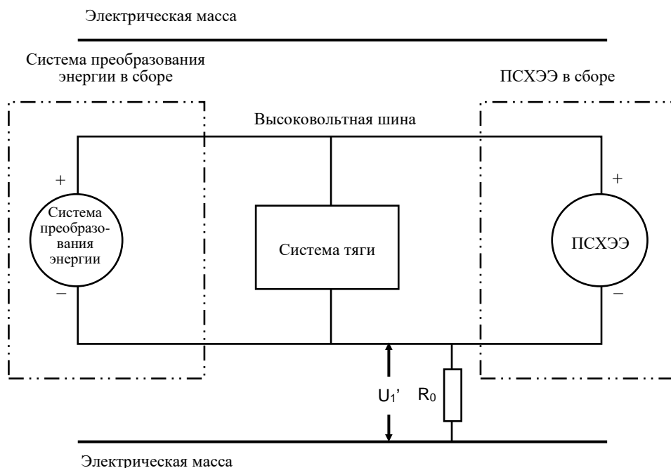
Рис. 5 Измерение U_1'
