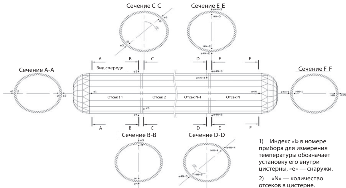
Рис. 3 Схема размещения приборов для измерения температуры воздуха внутри и снаружи цистерны с тремя и более отсеками
