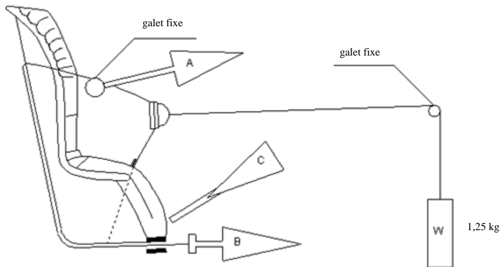
Figure 1 Conditionnement des tendeurs montés directement sur le système amélioré de retenue pour enfants
