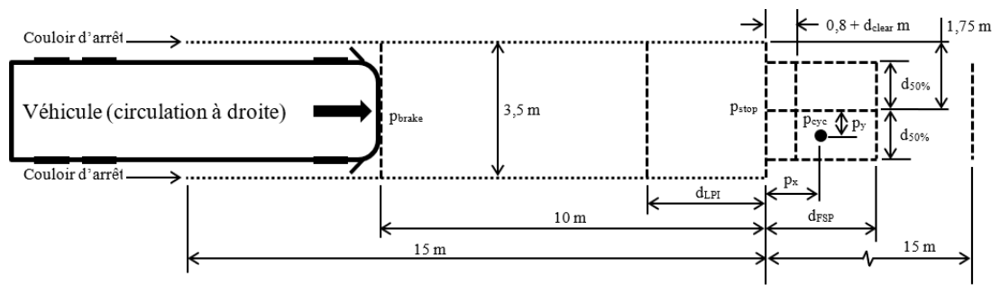
Figure 2 Configuration pour les essais longitudinaux avec cycliste
