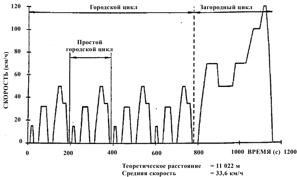
Рис. 1 Испытательный цикл НЕЕЦ
