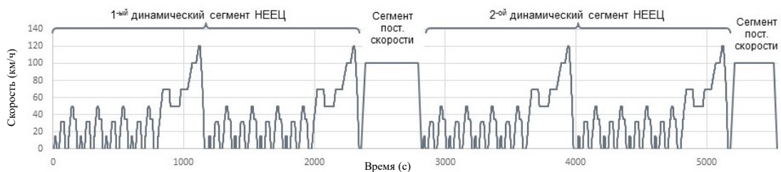
Сокращенная последовательность испытания НЕЕЦ
