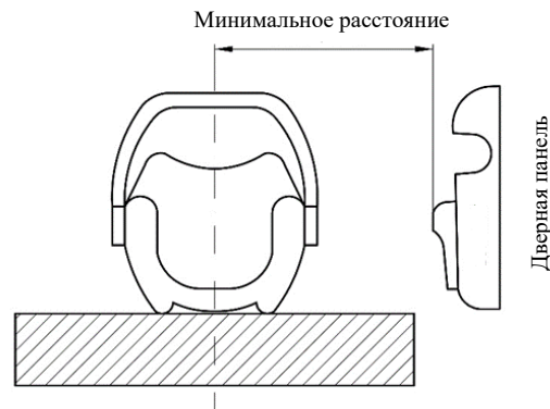
Рис. 3 Минимальное расстояние для бокового удара
