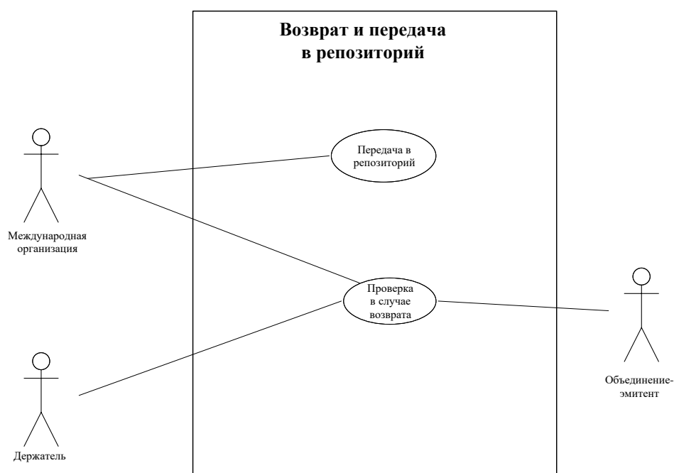
Диаграмма варианта использования процедуры возврата и передачи в репозиторий
