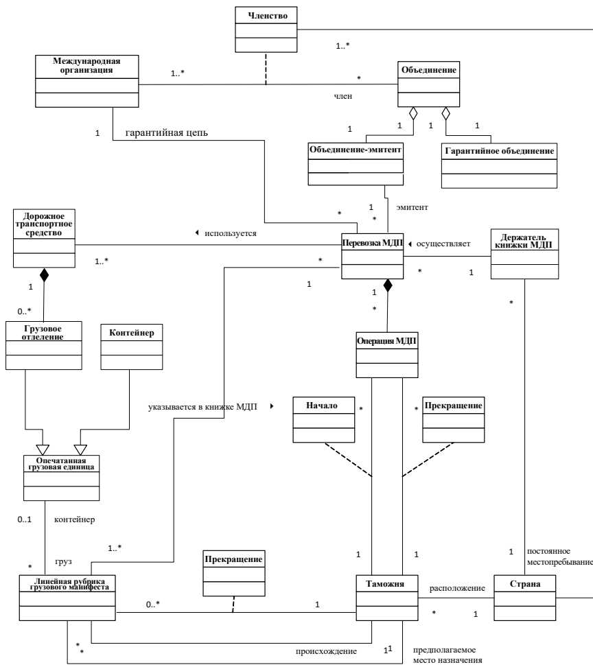
Высокоуровневая диаграмма классов
