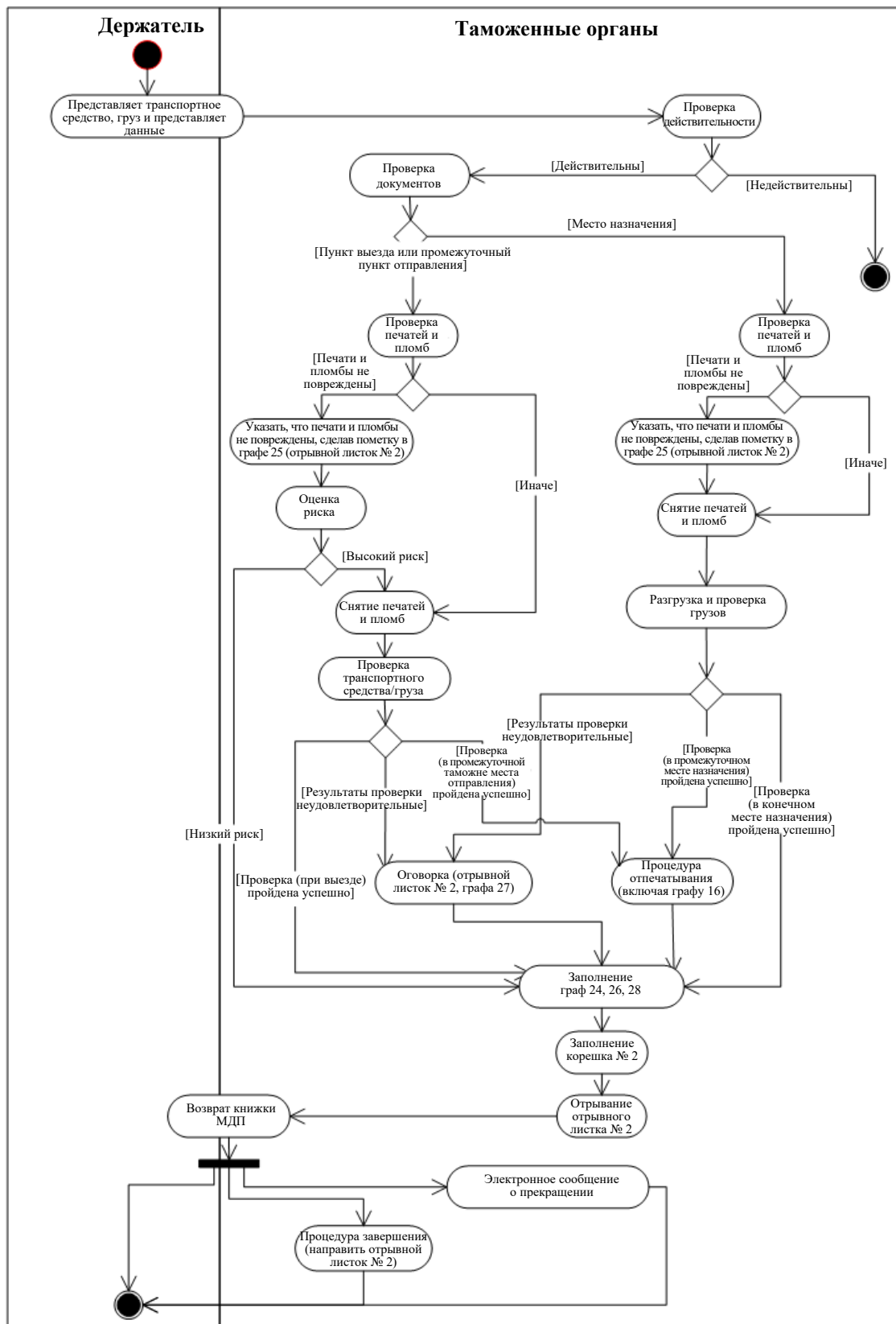
4.6.4 Структурное описание диаграммы деятельности при использовании процедуры прекращения операции МДП
