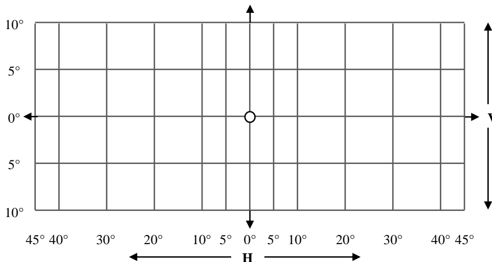
Figure A3-VII Répartition de la lumière pour les feux de position latéraux de la catégorie SM1
