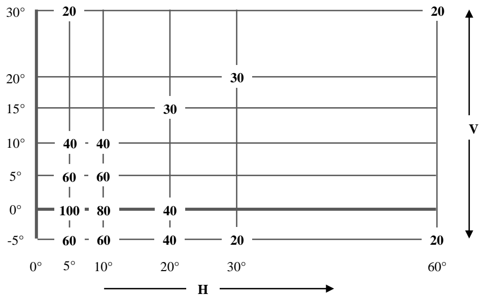
Figure A3-IV Répartition de la lumière pour les feux indicateurs de direction de la catégorie 6
