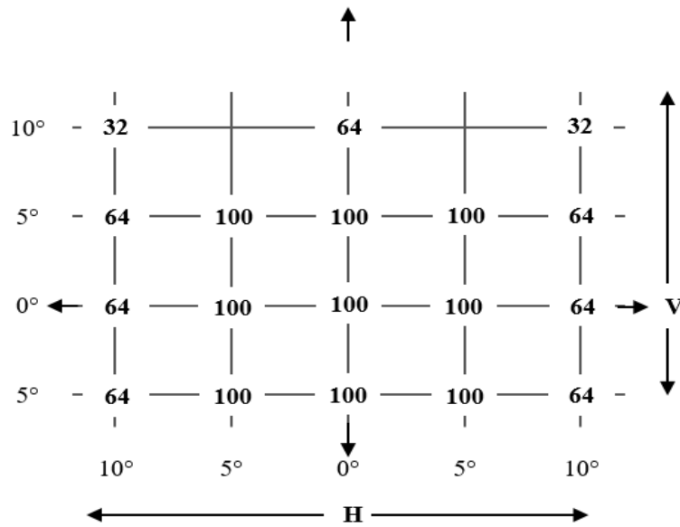
Figure A3-III Répartition de la lumière pour les feux stop des catégories S3 et S4
