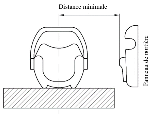
Figure 6 Distance minimale pour l'essai de choc latéral
