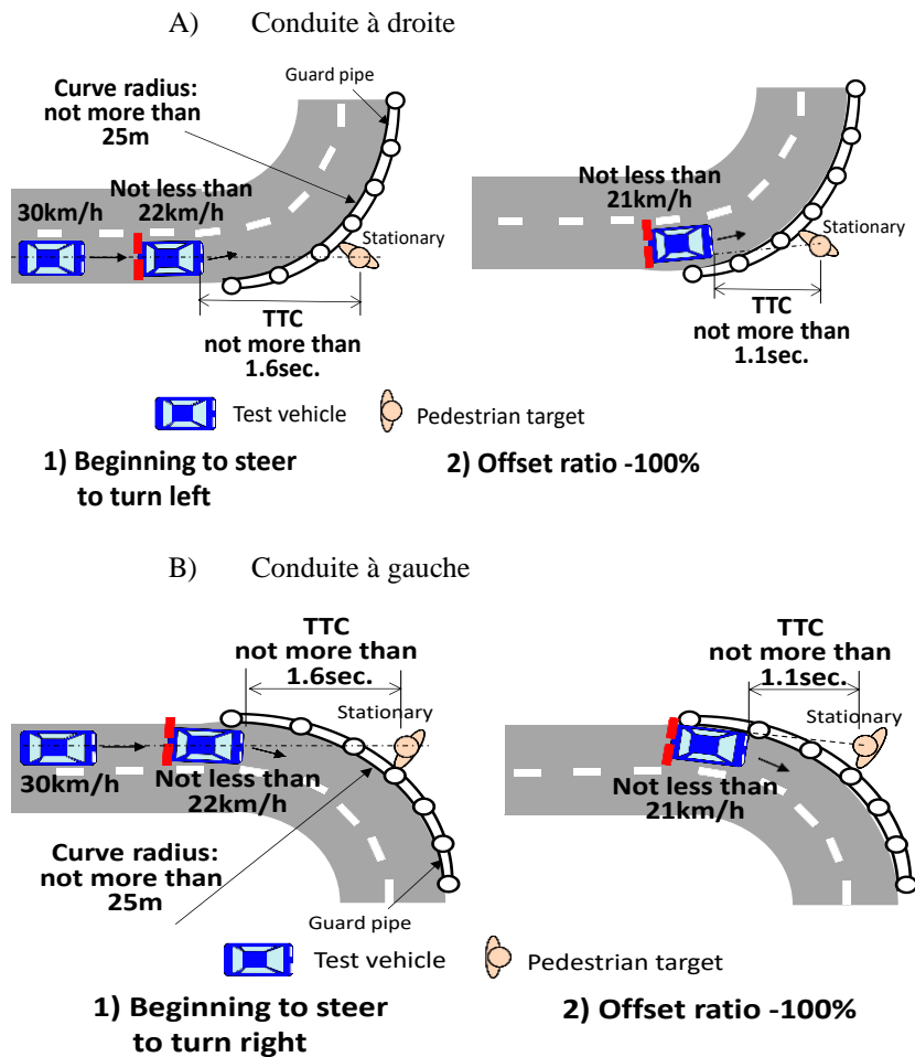
Figure 3 Virage équipé d'une glissière de sécurité et objet immobile
