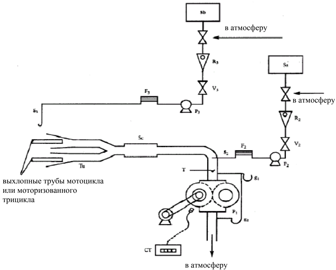
Рис. 6-2: Оборудование для отбора проб газов и измерение их объема
