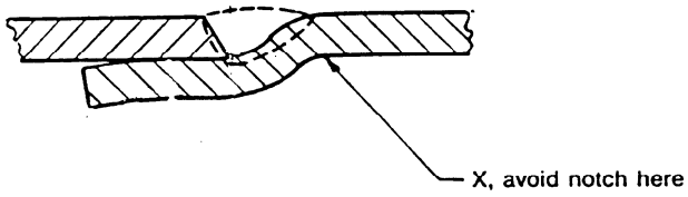
joggle weld
