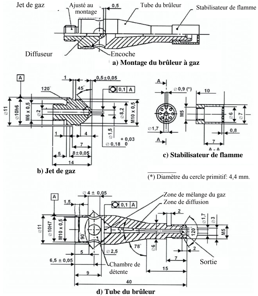
Figure 3 Brûleur à gaz (dimensions en millimètres)
