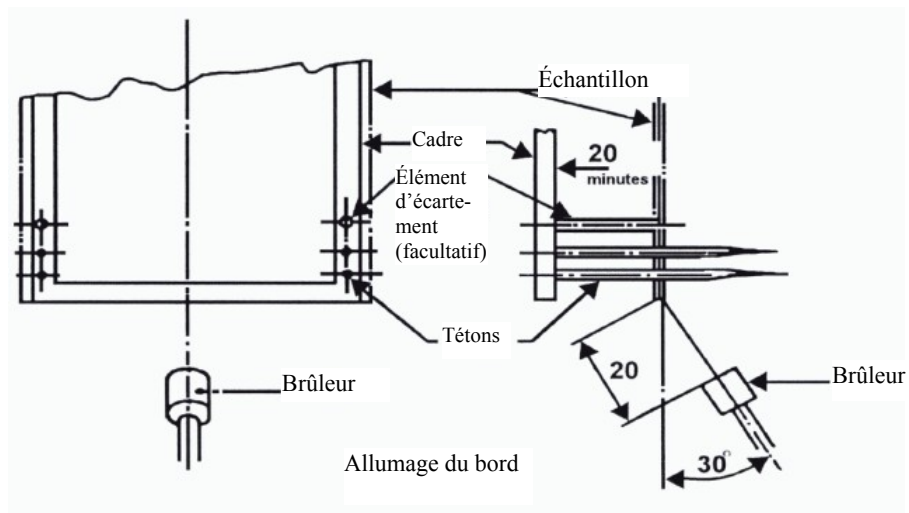
Figure 2 Emplacement du brûleur
