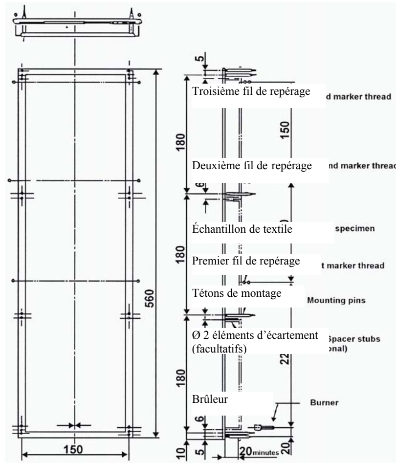
Figure 1 Porte-échantillon (dimensions en millimètres)
