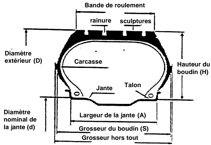
Figure explicative (voir paragraphes 2.2 et 4.1) Vue d'un pneumatique en coupe
