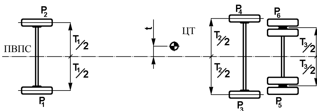
Рис. А3.2 - Положение центра тяжести в поперечной плоскости
