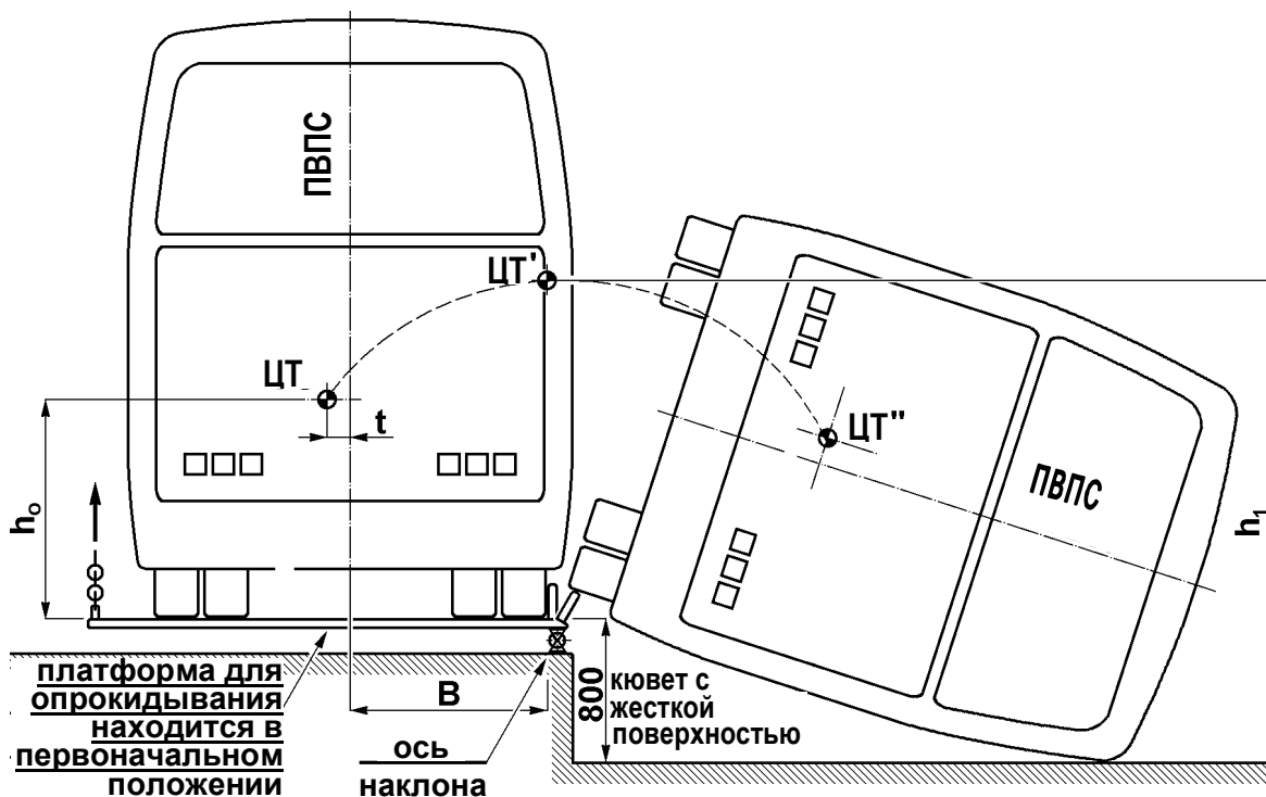
Рис. 3 - Испытание на опрокидывание комплектного транспортного средства с указанием траектории перемещения центра тяжести из первоначального положения неустойчивого равновесия
