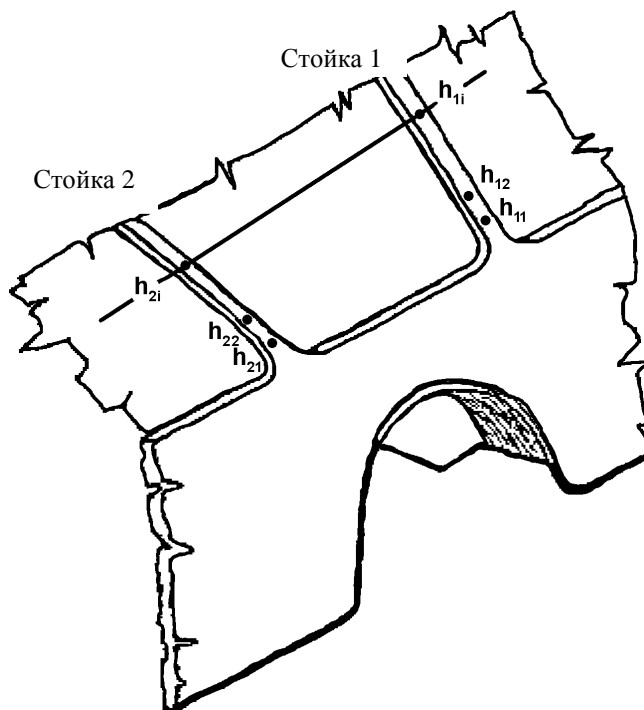
Рис. 1 - Определение контура деформированной конструкции
