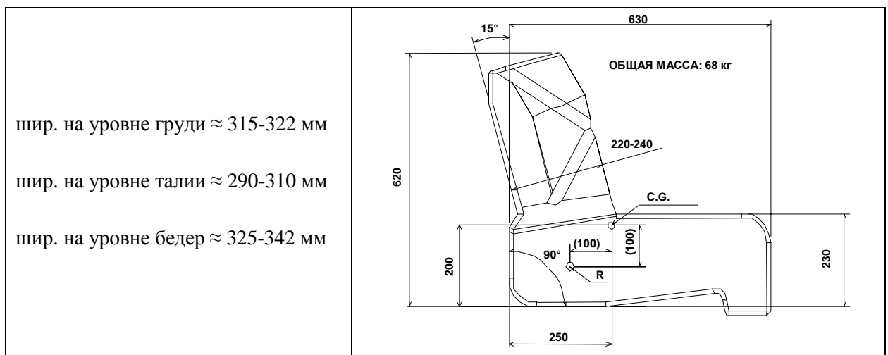
Рис. А5.2 - Размеры для антропоморфического балласта
