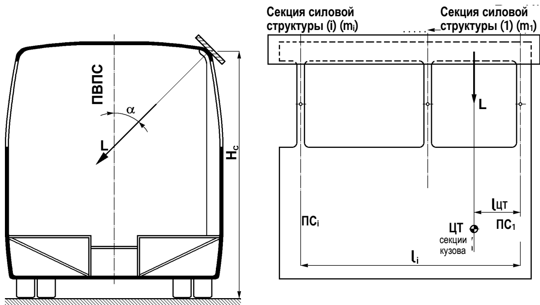
Рис. А7.1 - Применение нагрузки к секции кузова
