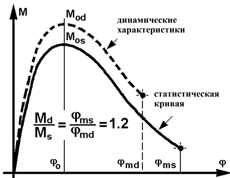
Рис. А8. 1А.2 - Динамические характеристики пластического шарнира, получаемые на основе статической кривой
