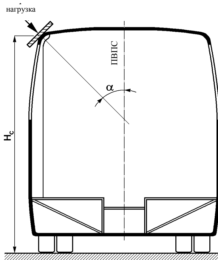
Рис. А8. 2 - Приложение нагрузки к верхней части силовой структуры
