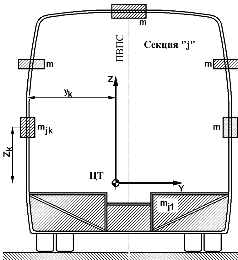
Рис А4.4 – Распределение массы в поперечном разрезе секции
