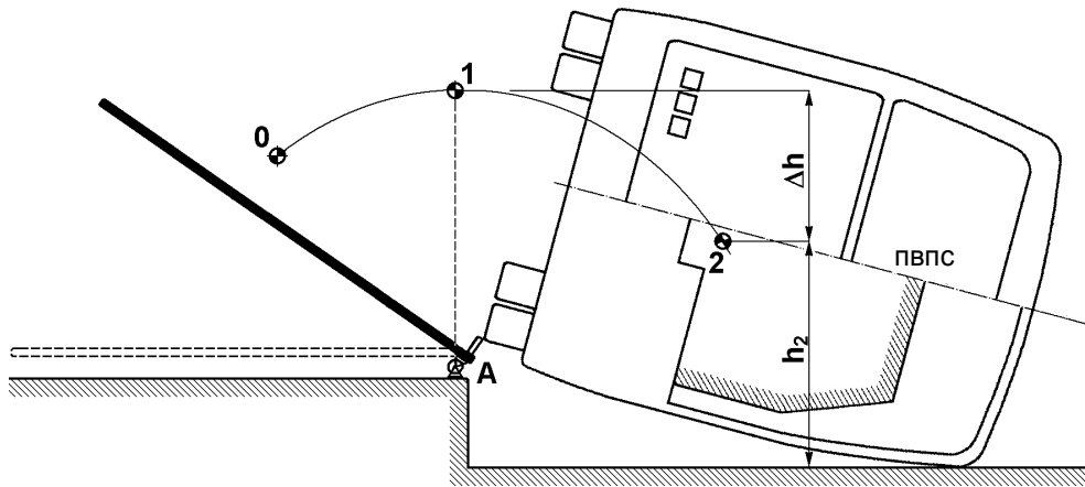
Рис. А7.А1.2 - Определение величины вертикального перемещения центра тяжести транспортного средства
