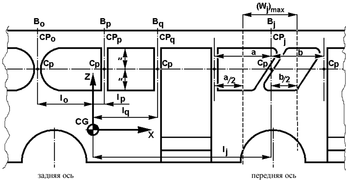
Рис. А4.2 - Определение длины секций силовой структуры
