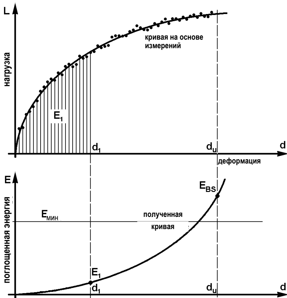
Рис. А7.2 - Энергия, поглощенная секцией кузова, в соответствии с основывающейся на измерениях кривой зависимости прогиба от нагрузки
