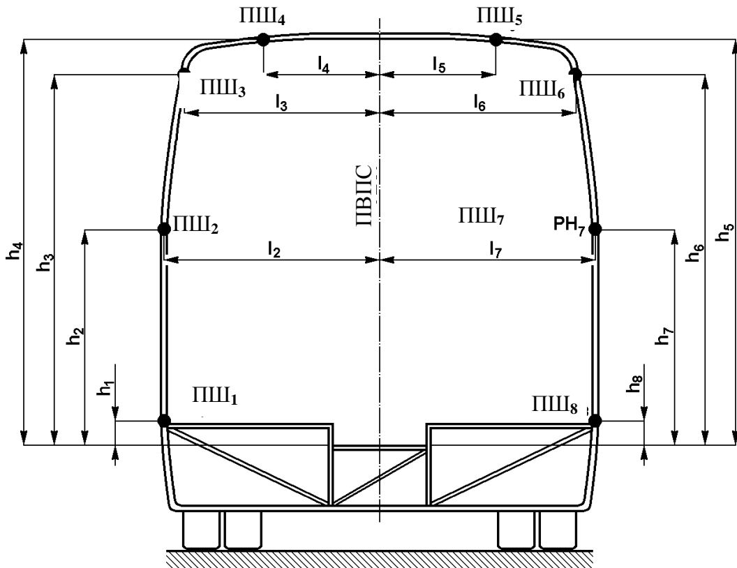
Рис. А8. 1 - Геометрические параметры пластических шарниров на секции силовой структуры
