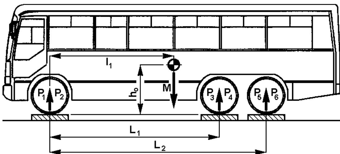
Рис. А3.1 - Положение центра тяжести в продольной плоскости
