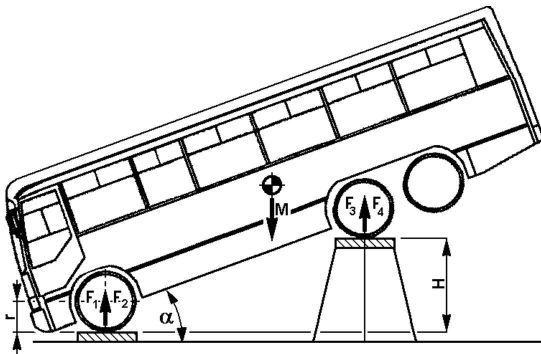
Рис. А3.3 - Определение высоты центра тяжести
