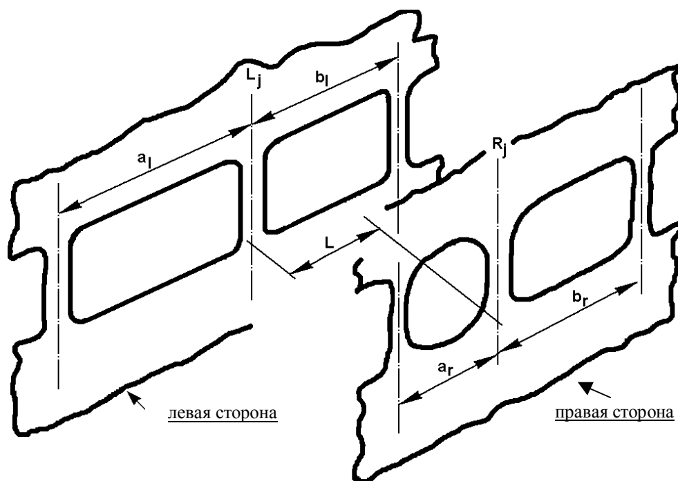
Рис. А4.3 - Определение длины секции в том случае, когда стойки с каждой стороны секции не находятся в одной и той же поперечной плоскости
