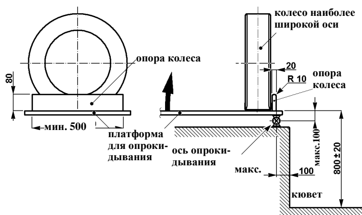
Рис. А5.1 – Геометрические характеристики устройства для опрокидывания
