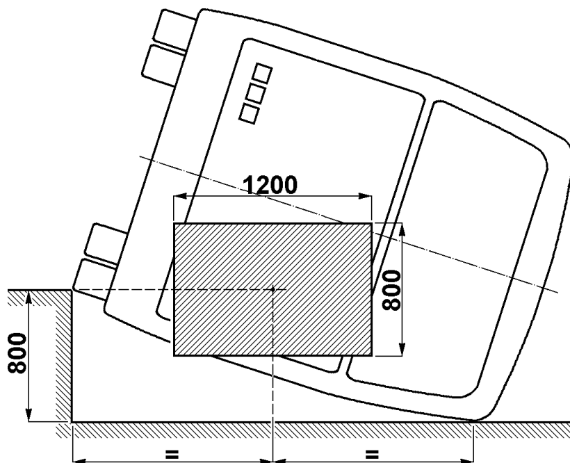
Рис. А5.3а - Рекомендуемая зона обзора для внешнего фотоаппарата
