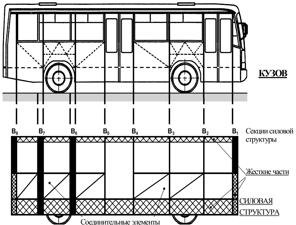
Рис. А4.1 - Определение силовой структуры по кузову
