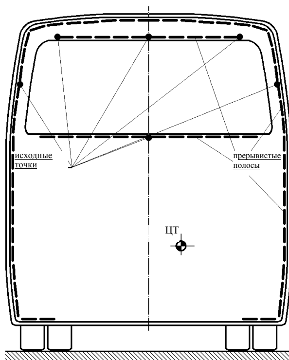
Рис. А5.3б - Рекомендуемое обозначение положения центра тяжести и контура транспортного средства
