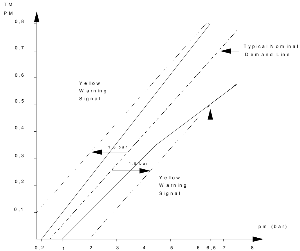
D I A G R A M 2 . T r a c t i v e U n i t s f o r S e m i - t r a i l e r s .
