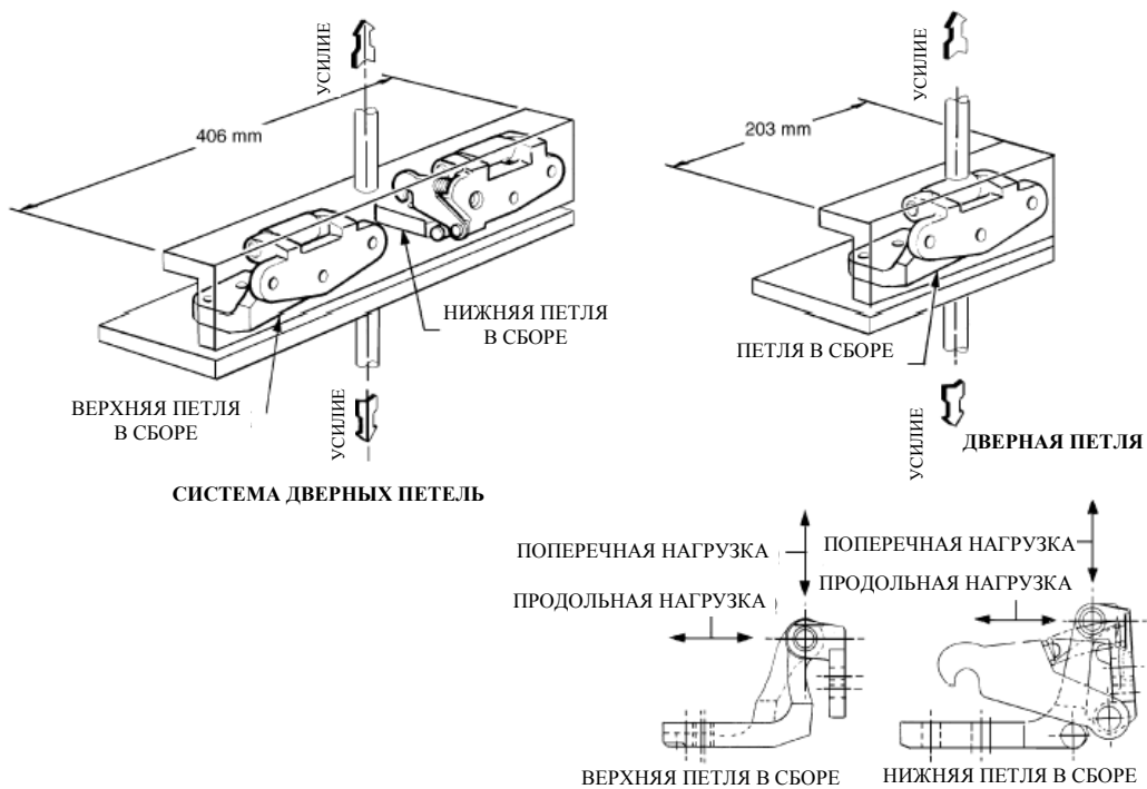
Рис. 5-1 - Арматуры для статических испытаний
