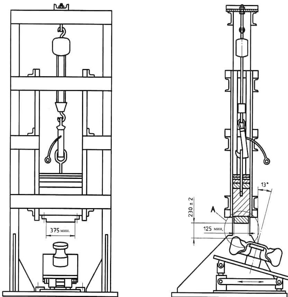
Рис. 1 - Установка для испытания на нагрузку при ударе
