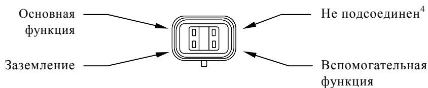
Рис. 2 – Схема разъема
