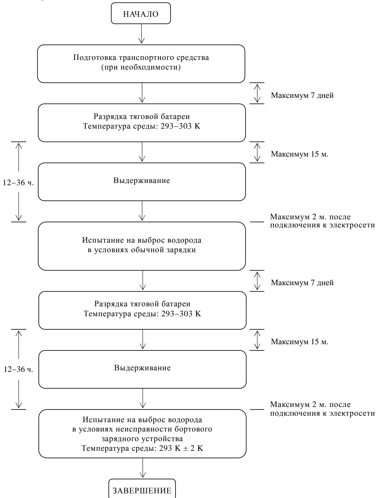
Рис. 1 Определение уровня выбросов водорода в процессе зарядки тяговой батареи
