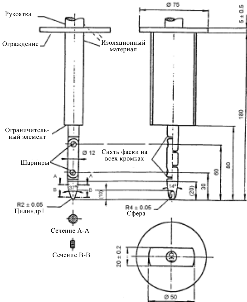
Рис. 1 Шарнирный испытательный штырь
