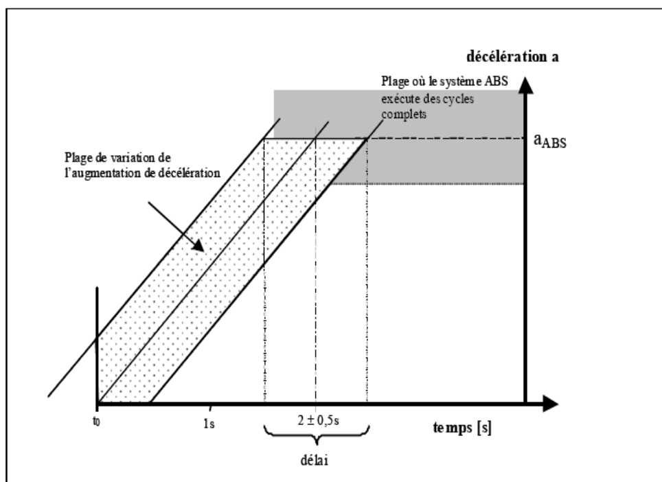
Plage de décélération pour la détermination de F_{ABS} et a_{ABS}
