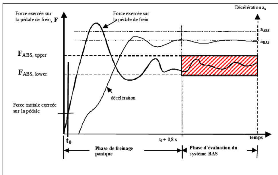
Figure 2 Essai 2 d'un système BAS de catégorie «B»
