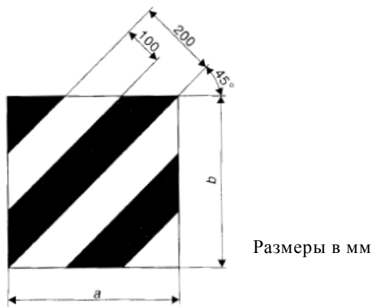
Рис. 2 Сигнальная табличка или сигнальная наклейка
