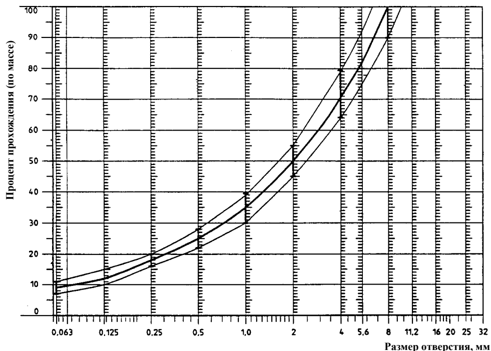
Рис. 2 Гранулометрическая кривая, отражающая состав скелетного материала асфальтобетонной смеси, с допусками
