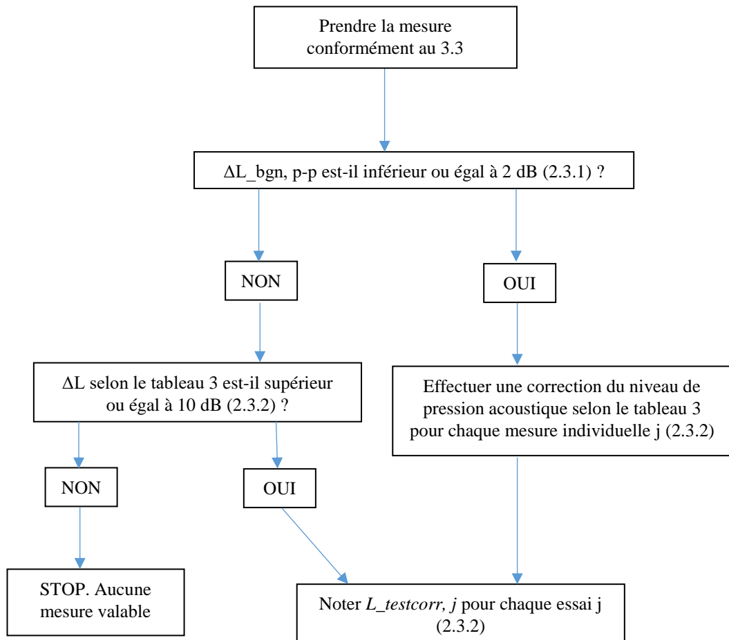
Figure 5 Critères de correction des mesures du niveau de pression acoustique pondéré A du véhicule
