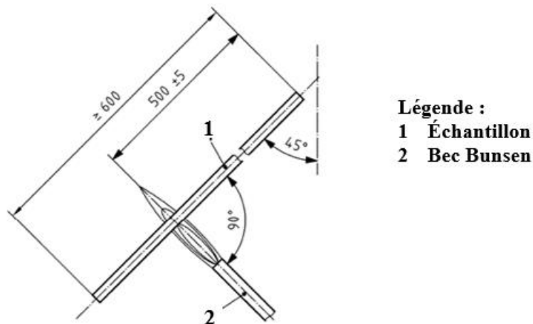
Figure 1 Appareillage de mesure de la résistance à la propagation des flammes (dimensions en millimètres)
