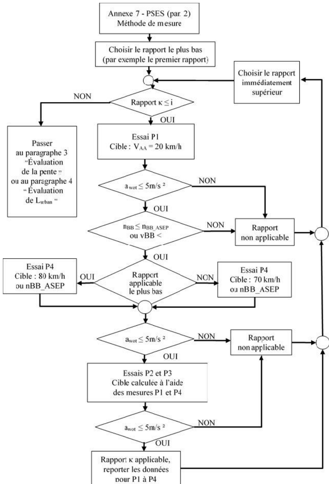
Figure 3 Diagramme de détermination des points d'essai P_j conformément au paragraphe 2 de l'annexe 7, "Méthode de mesure"
