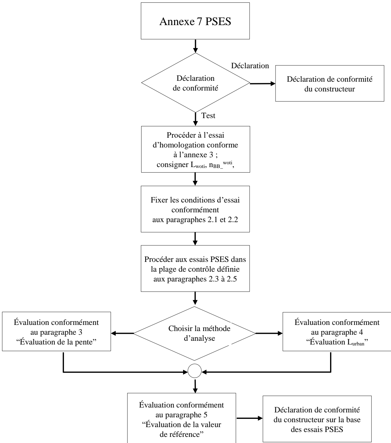
Diagramme de la méthode d'évaluation pour les PSES selon l'annexe 7
