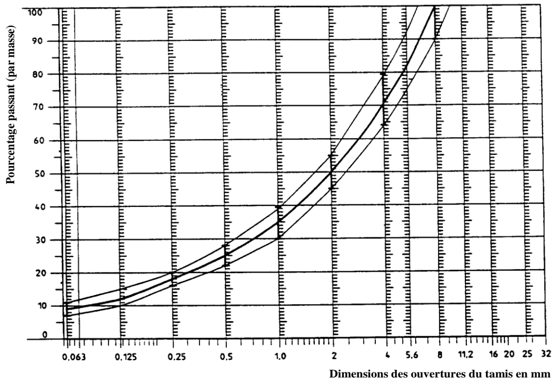
Figure 2 Courbe granulométrique des granulats enrobés, avec tolérances
