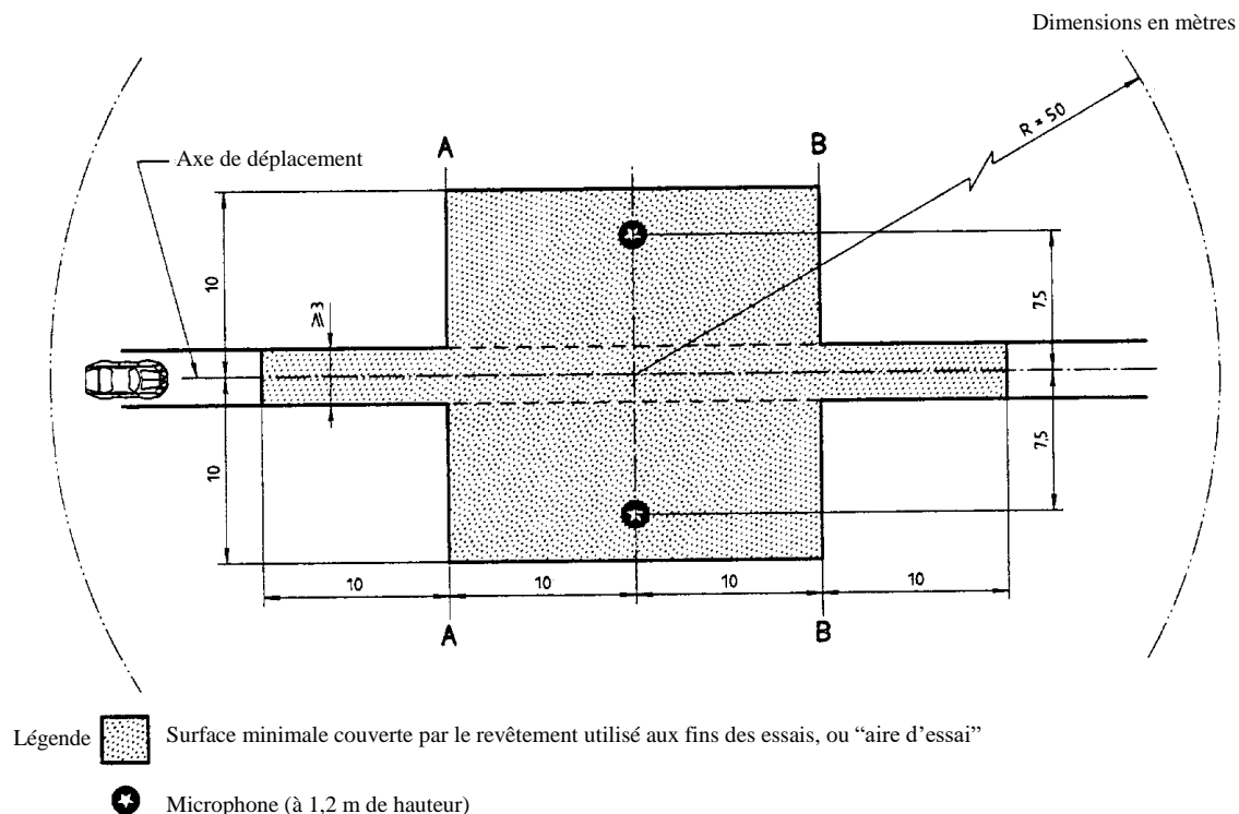
Figure 1 Prescriptions minimales concernant l'“aire d'essai” (zone ombrée)
