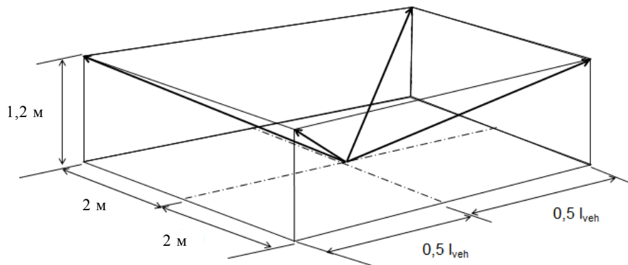
Рис. 3 Минимальные допустимые габариты полубезэховой камеры
