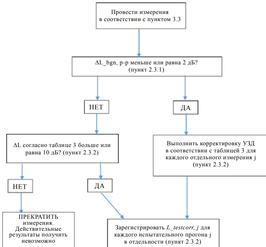
Рис. 5 Критерии корректировки измеренного значения взвешенного по шкале А уровня звукового давления транспортного средства
