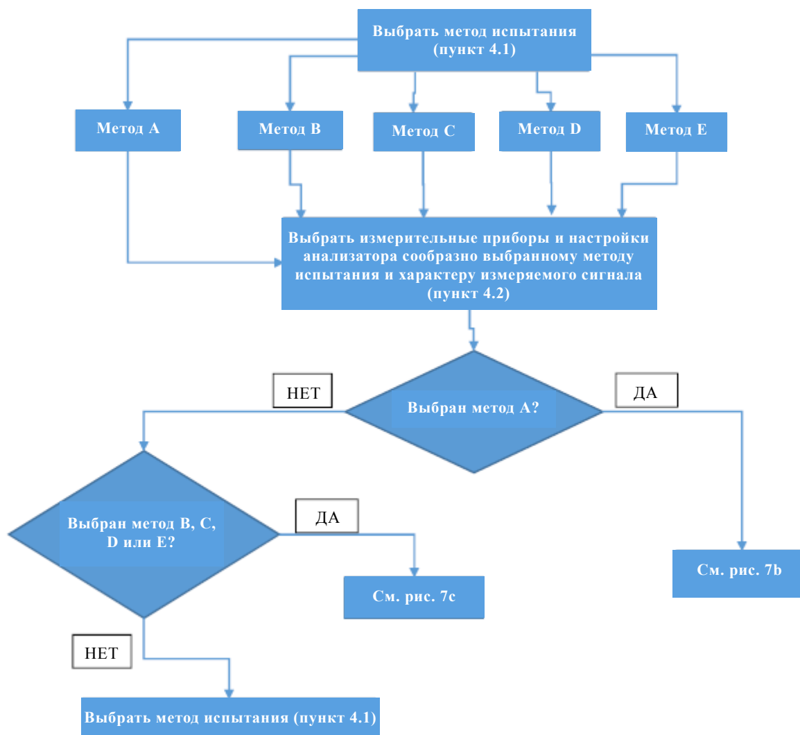
Рис. 7а Процедуры испытания для измерения сдвига частоты
