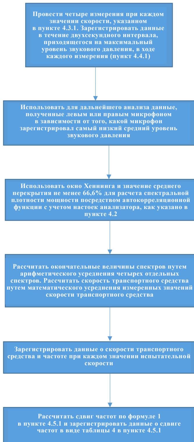
Рис. 7b Процедуры испытания для измерения сдвига частоты методом А
