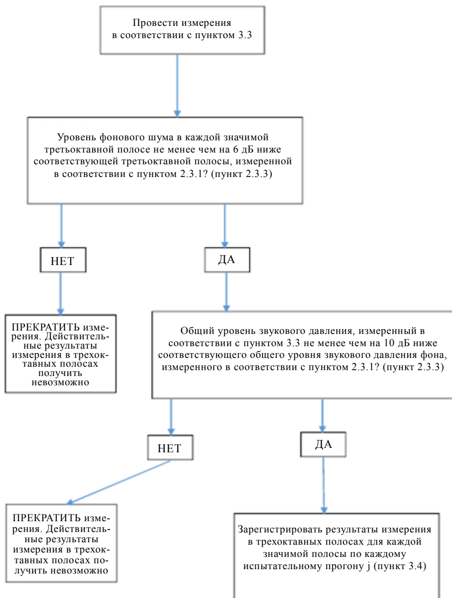
Рис. 6 Требования в отношении фонового шума для анализа в третьоктавных полосах
