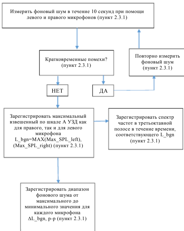
Рис. 4 Определение диапазона фонового шума
