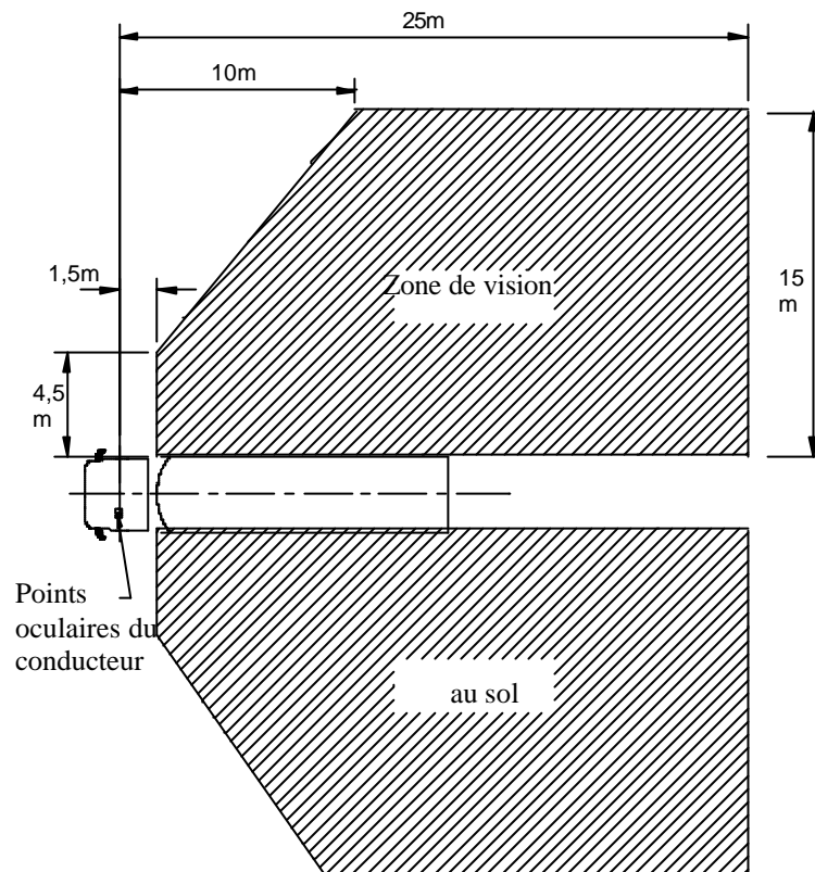
Figure 6 : Champ de vision d'un rétroviseur "grand angle" de la classe IV
