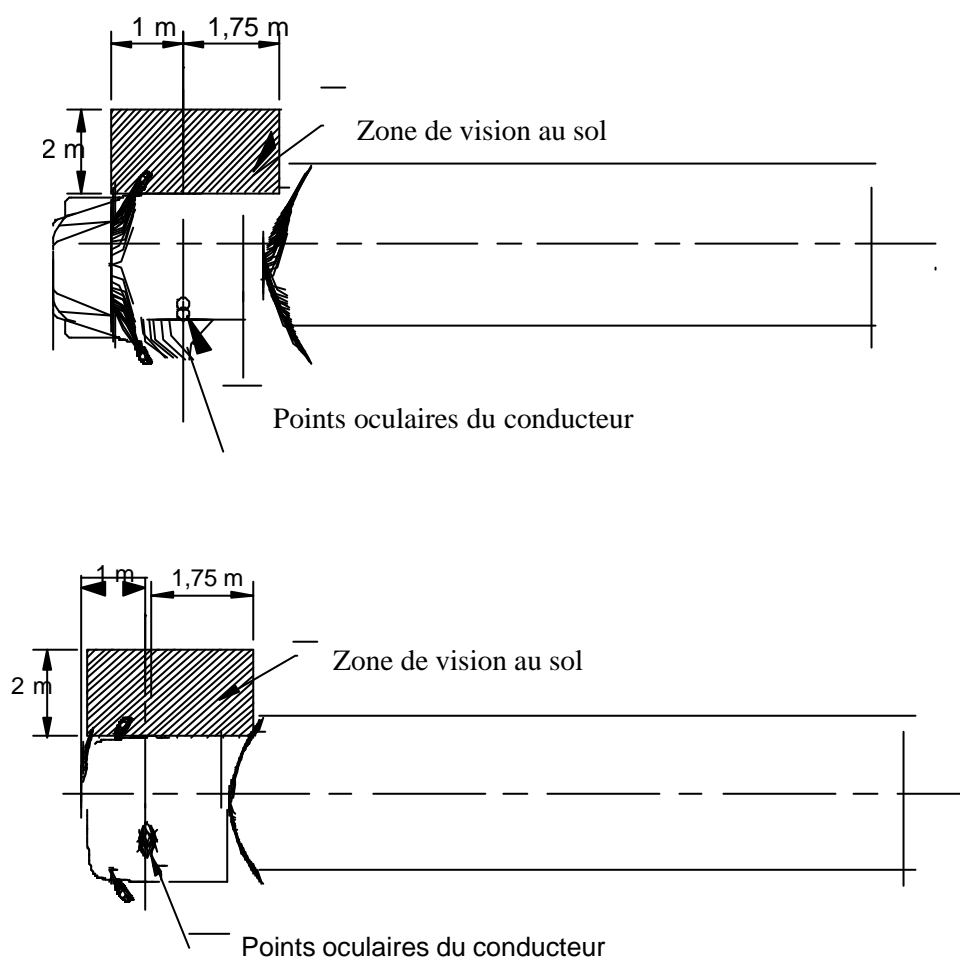
Figures 7 a) et 7 b): Champ de vision d'un rétroviseur "d'accostage" de la classe V
