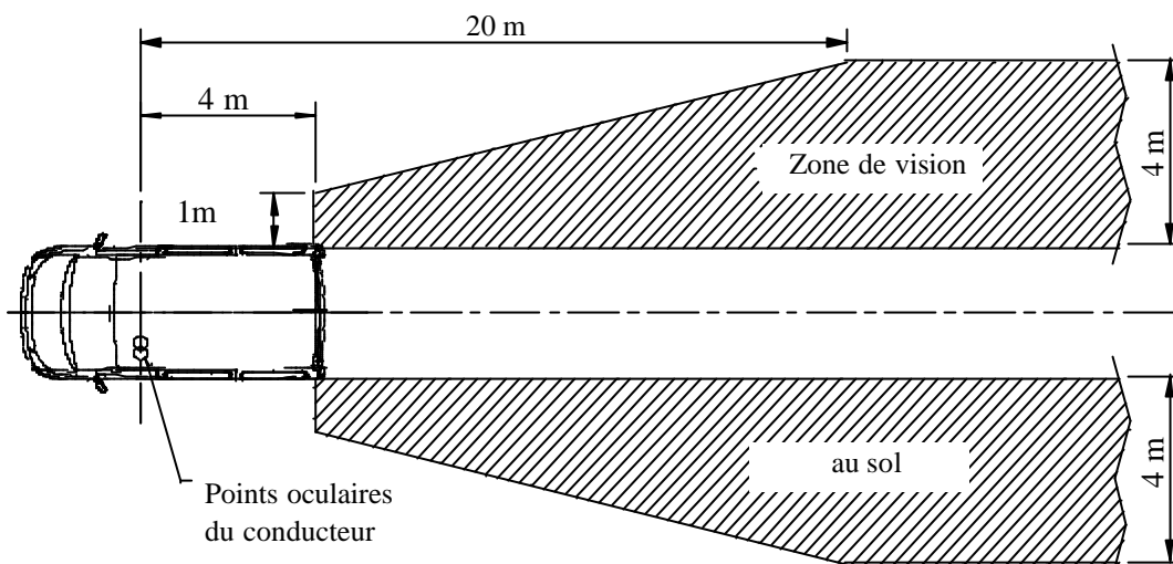
Figure 5 : Champ de vision d'un rétroviseur de la classe III
