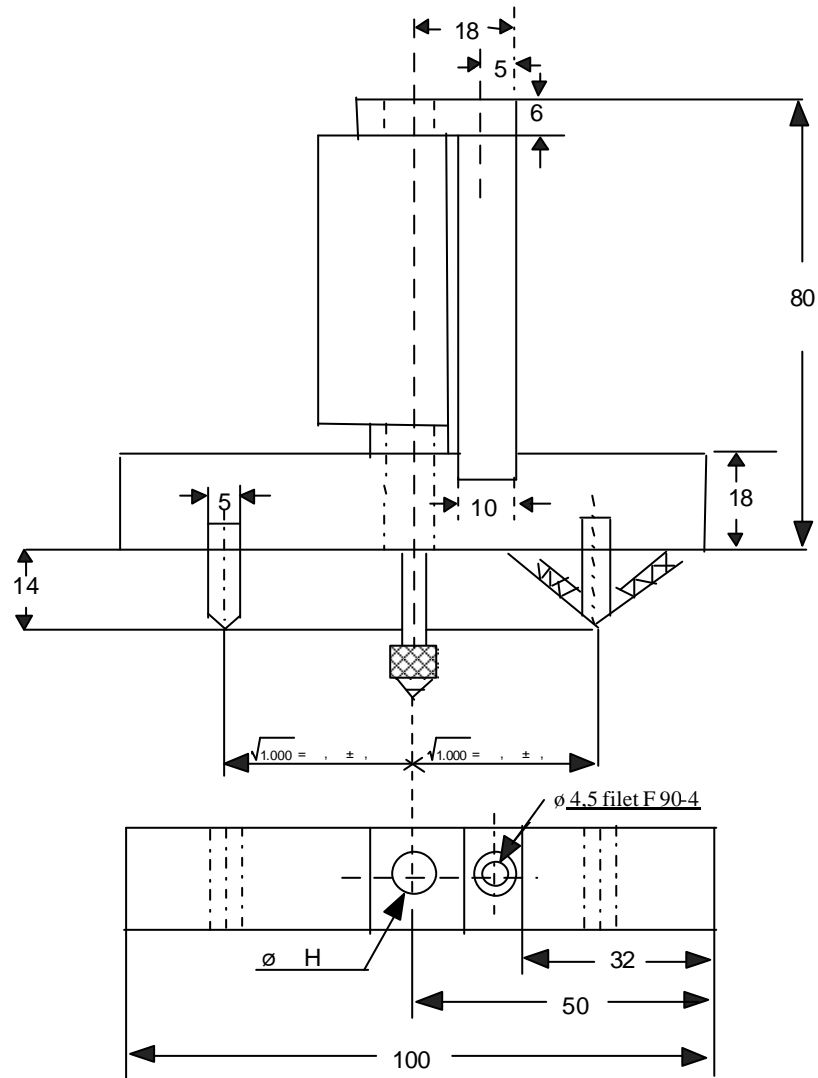
Figure 1: Sphéromètre
