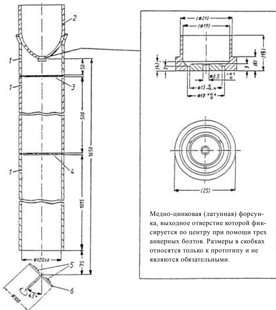
Устройство для испытания под воздействием струи песка
