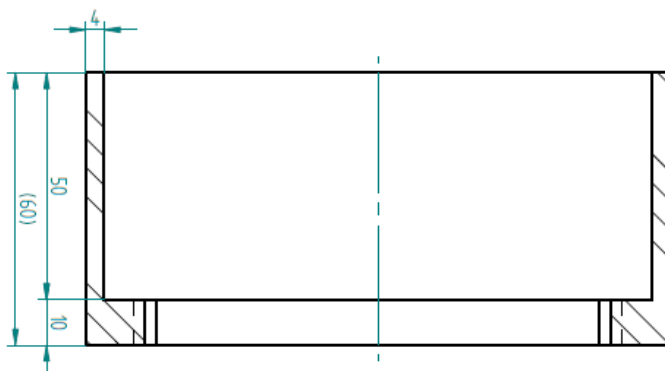
Рис. 2 Вид проекции А в разрезе
