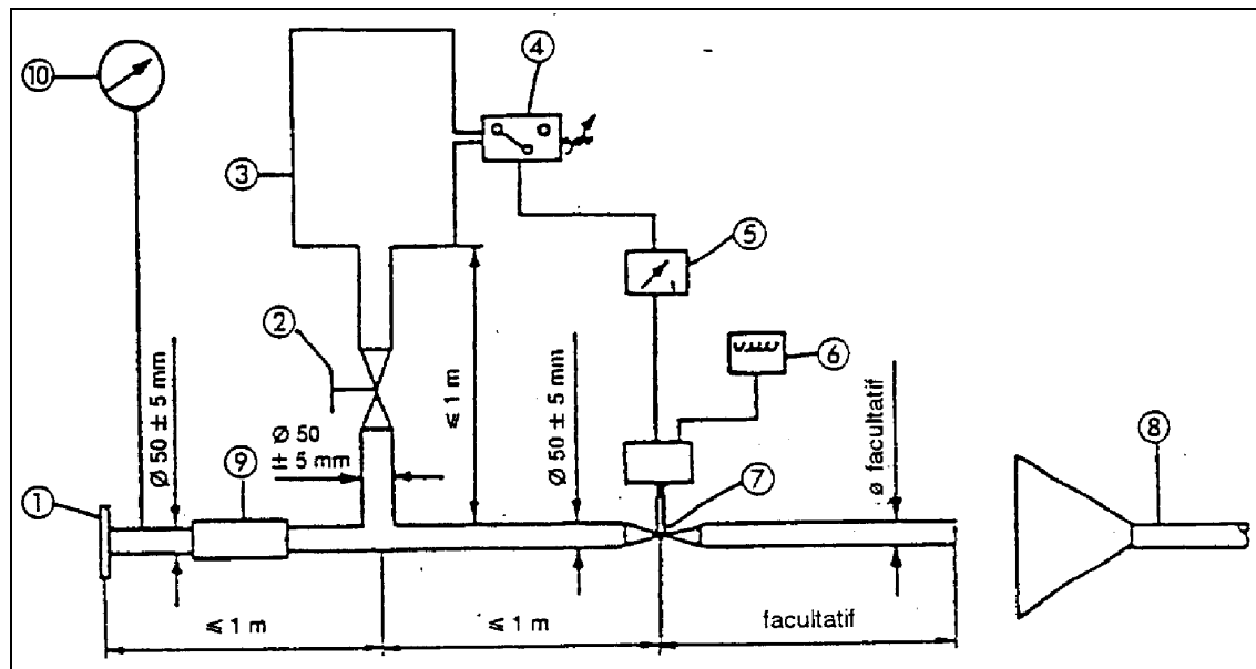
Figure 3 Appareillage d'essai de conditionnement par pulsions
