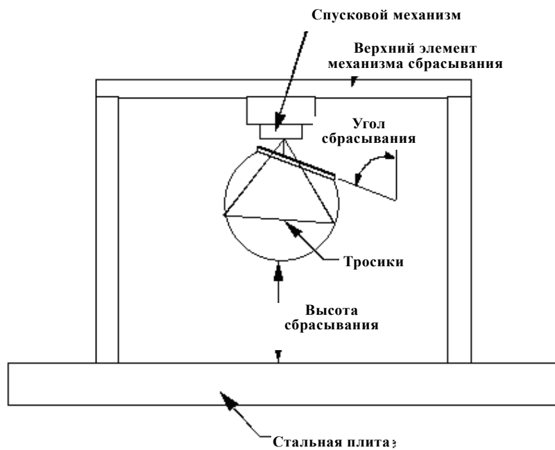
Рисунок 8 Испытательная установка для проведения динамического испытания ударного элемента в виде модели головы на соответствие биомеханическим характеристикам
