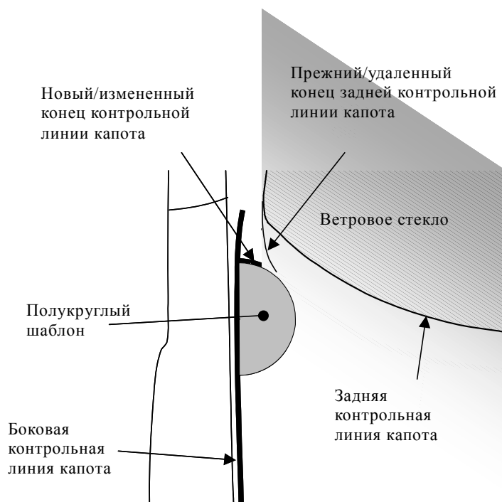
Рисунок 4 Определение точки пересечения задней и боковой контрольных линий капота
