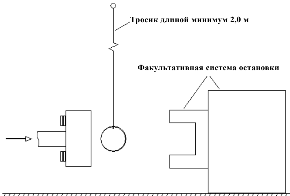
Рисунок 8 Испытательная установка для проведения динамического испытания ударного элемента в виде модели головы на соответствие биомеханическим характеристикам
