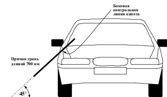
Рисунок 9 Боковая контрольная линия
