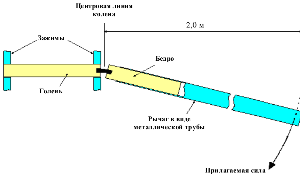
Рисунок 3 Вид сверху на испытательную установку для проведения статического испытания ударного элемента в виде модели нижней части ноги на изгиб в целях сертификации
