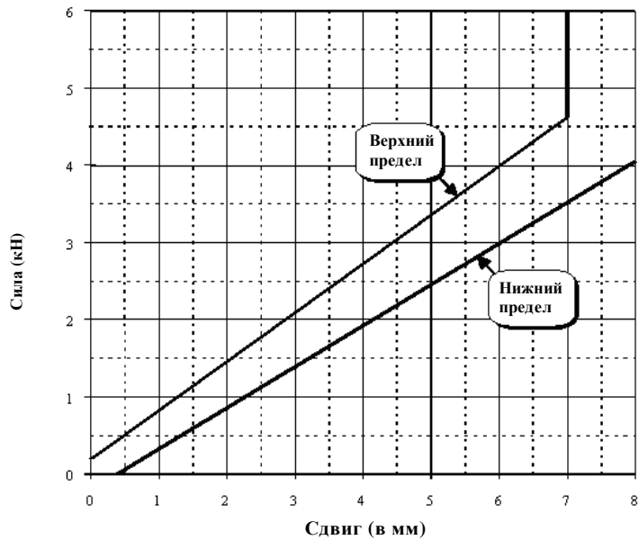
Рисунок 2 Требование к зависимости величины сдвига от силы в ходе статического испытания ударного элемента в виде модели нижней части ноги на сдвиг в целях сертификации
