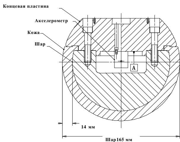
Рисунок 4 Ударный элемент в виде модели головы взрослого
