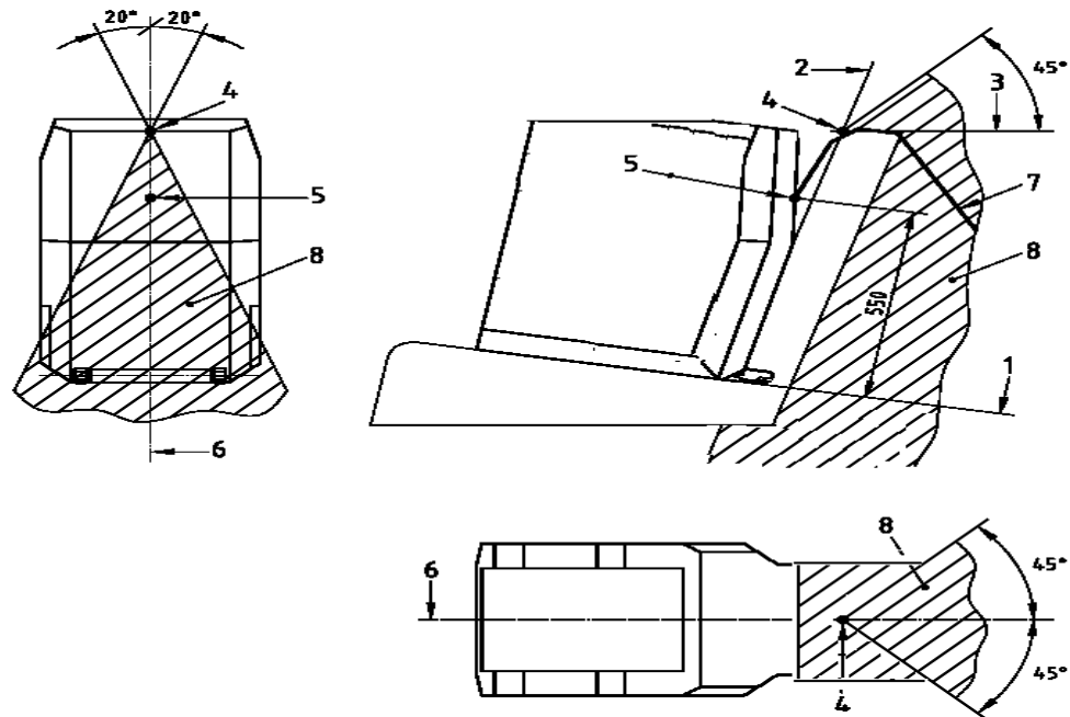
Рис. 11: Альтернативный метод размещения креплений верхней лямки с использованием зажимного приспособления "ISO/F2" (B); зона ISOFIX - вид сбоку, сверху и сзади
