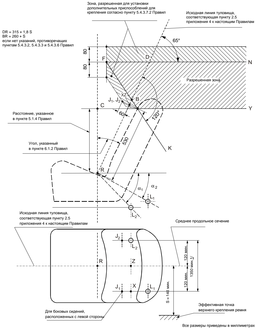
Рис. 1: Зоны расположения точек эффективного крепления ремня (На рисунке показан пример фиксирования верхнего крепления на боковой панели кузова)
