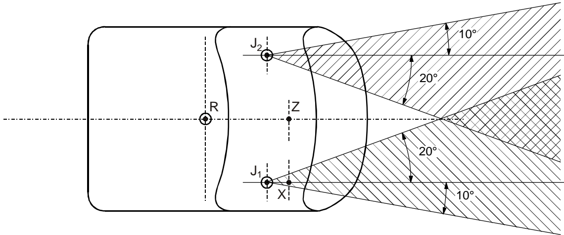
Рис. 2: Верхние точки эффективного крепления ремня, соответствующие пункту 5.4.3.7.3 Правил
