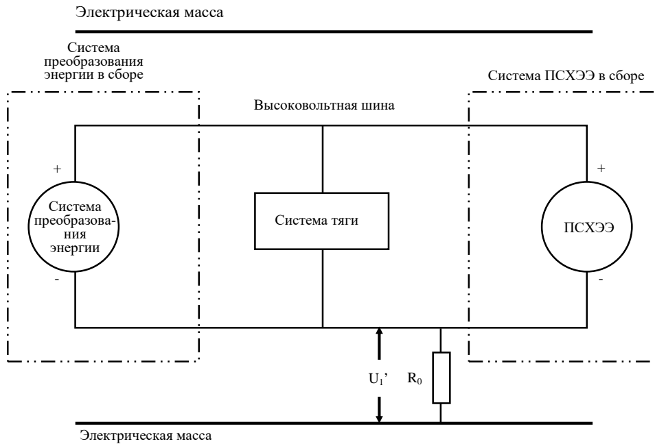
Рис. 5 Измерение U_1'
