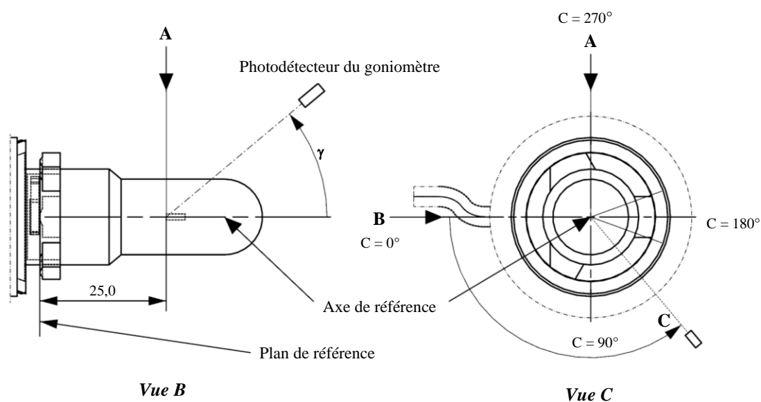
Figure 6 : Montage permettant de mesurer la répartition de l'intensité lumineuse et définition des plans C et de la direction \gamma
