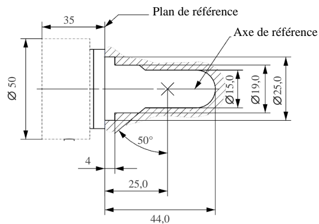
Figure 2 : Encombrement maximal 3/
