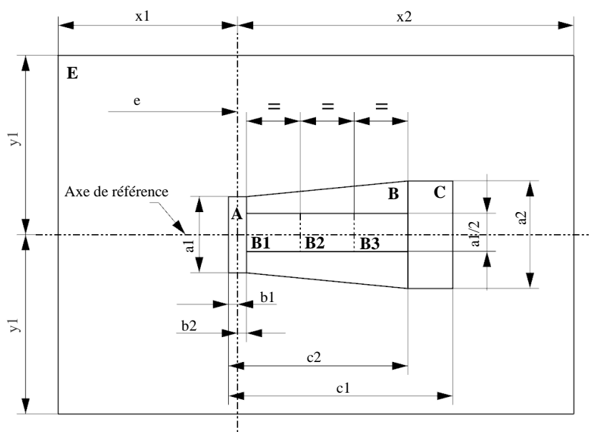
Figure 4 : Définition de la zone d'émission de lumière au moyen du gabarit (dimensions indiquées dans le tableau 2)
