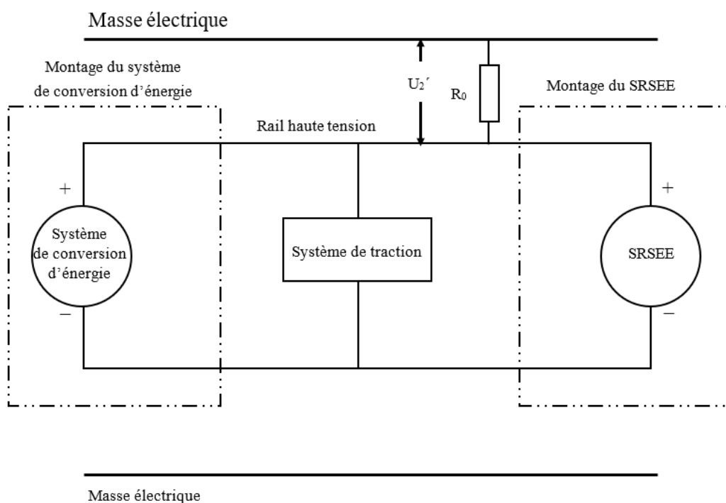
Figure 6 Mesure de U_2'
