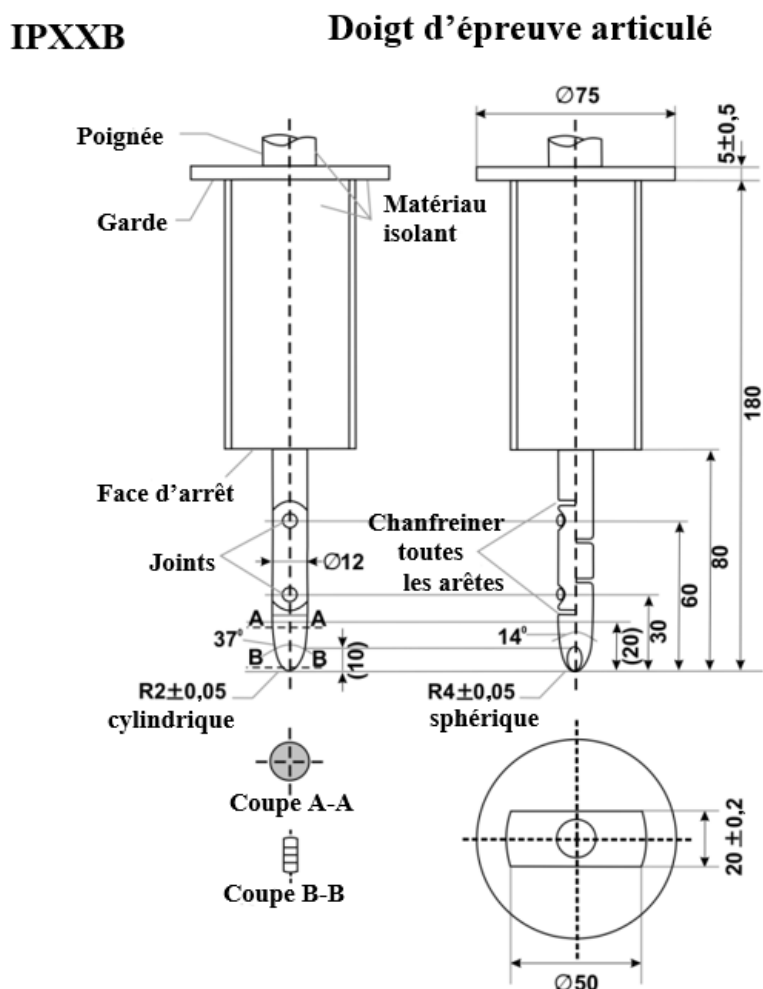
Figure 3 Doigt d'épreuve articulé
