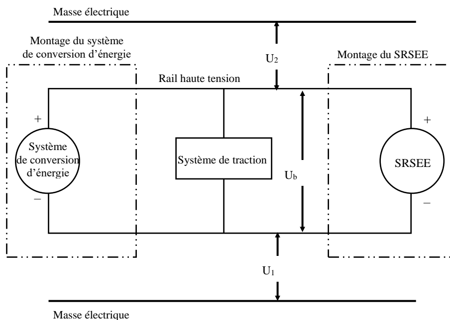
Figure 1 Mesure de U_b , U_1 et U_2
