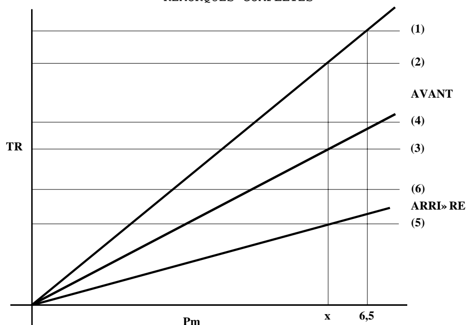
GRAPHIQUE DE CONTRÔLE POUR LE PARAGRAPHE 3.2.1.7 - REMORQUES COMPLÈTES
