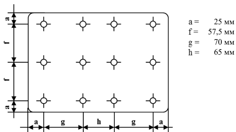
Рис. А3-XI: Точки измерения для таблички размером 255 x 165 мм
