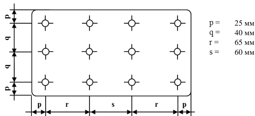
Рис. А3-ХIV: Точки измерения для таблички размером 240 x 130 мм
