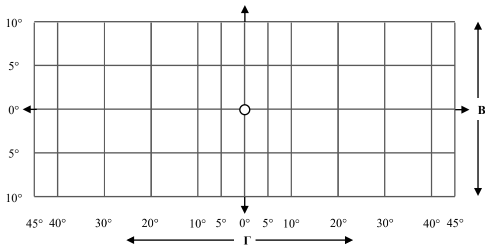
Рис. А3-VII: Распределение света боковых габаритных огней категории SM1
