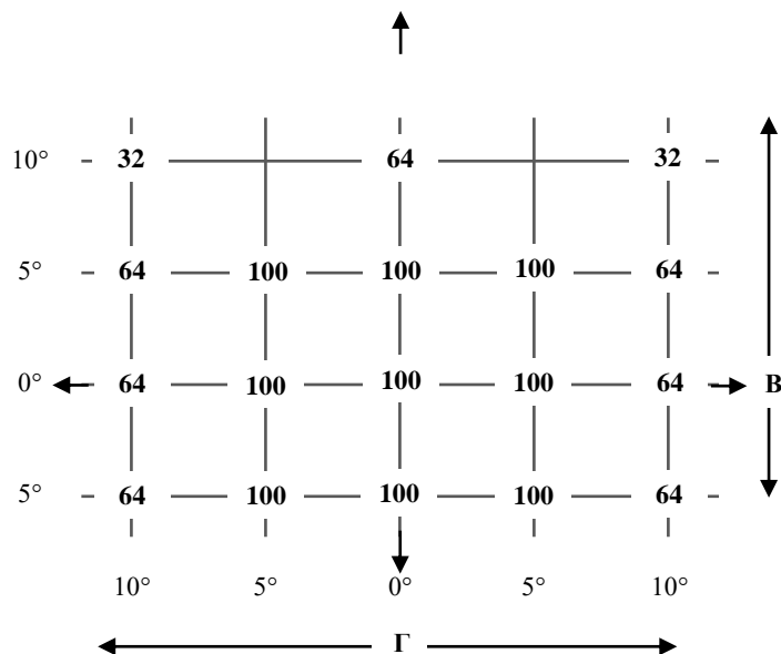
Рис. А3-III: Стандартное распределение света стоп-сигналов категорий S3 и S4
