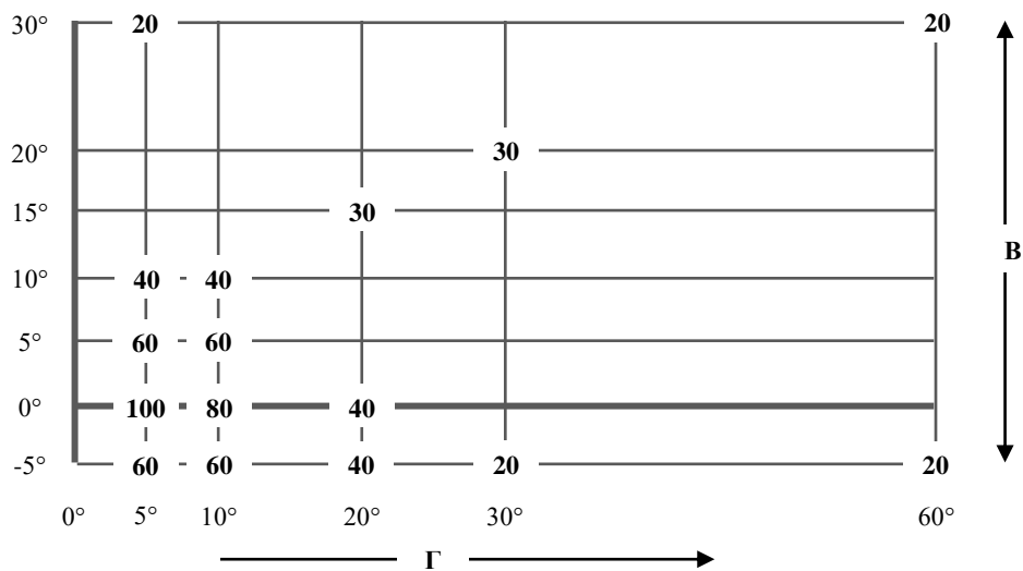
Рис. А3-IV: Распределение света огней указателей поворота категории б
