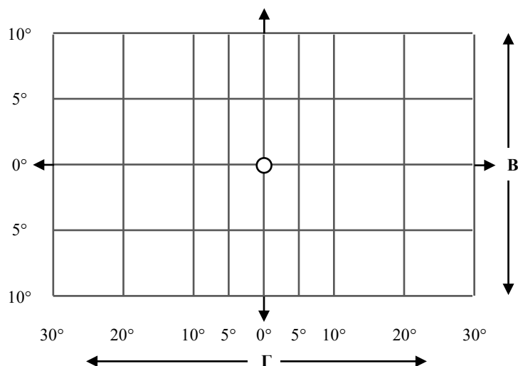
Рис. А3-VIII: Распределение света боковых габаритных огней категории SM2
