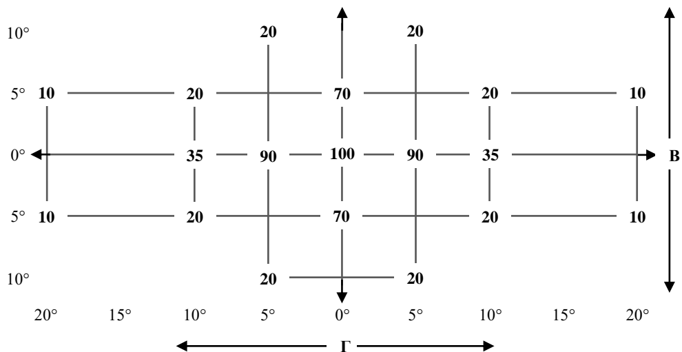
Рис. А3-I: Стандартное распределение света габаритных, стояночных, контурных огней, стоп-сигналов и указателей поворота
