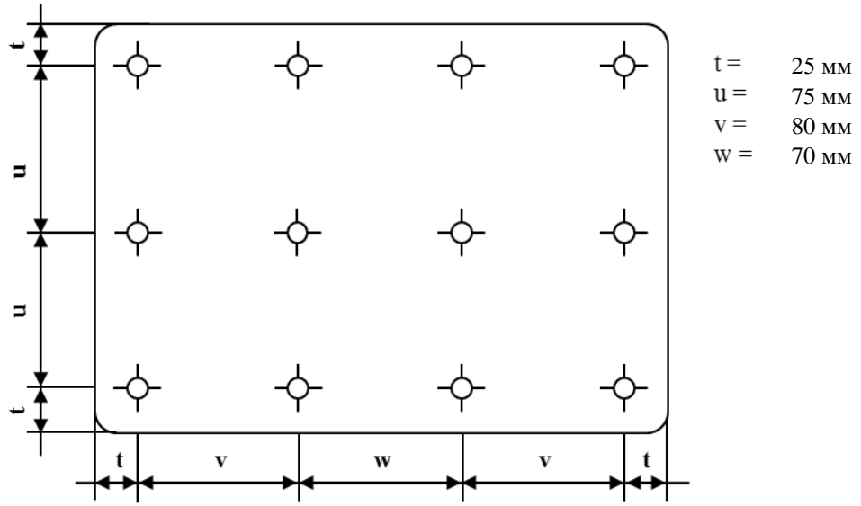
Рис. А3-ХV: Точки измерения для таблички размером 280 x 200 мм
