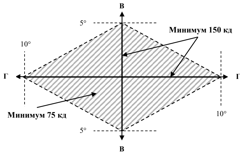
Рис. А3-VI Распределение света задних противотуманных огней
