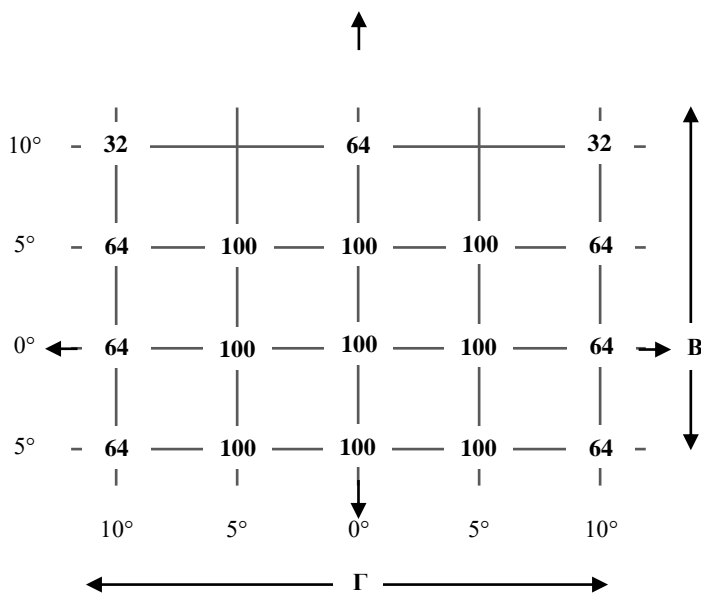
Рис. А3-III Стандартное распределение света сигналов торможения категорий S3 и S4
