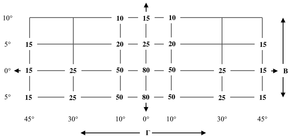
Рис. А3-V Распределение света огней заднего хода
