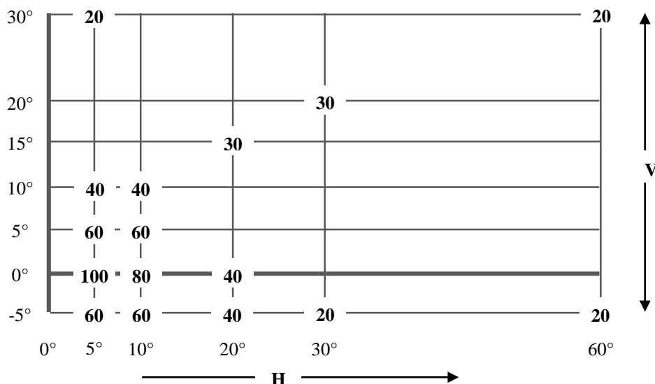
Figure A3-IV Répartition de la lumière pour les feux indicateurs de direction de la catégorie 6
