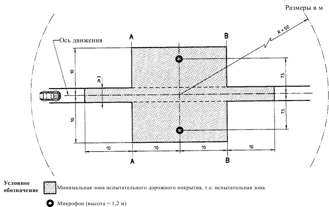
Рис. 1 Минимальные требования в отношении зоны с испытательным покрытием. Затемненная часть называется «испытательной зоной»
