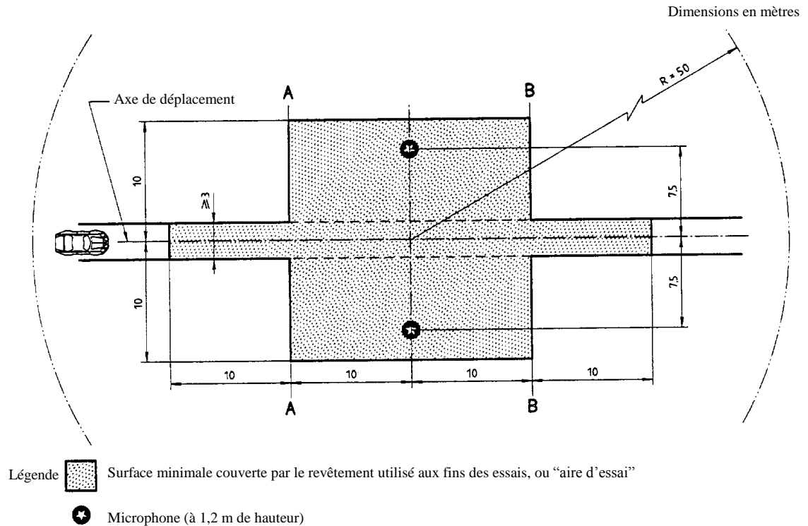
Figure 1 Prescriptions minimales concernant l'“aire d'essai” (zone ombrée)
