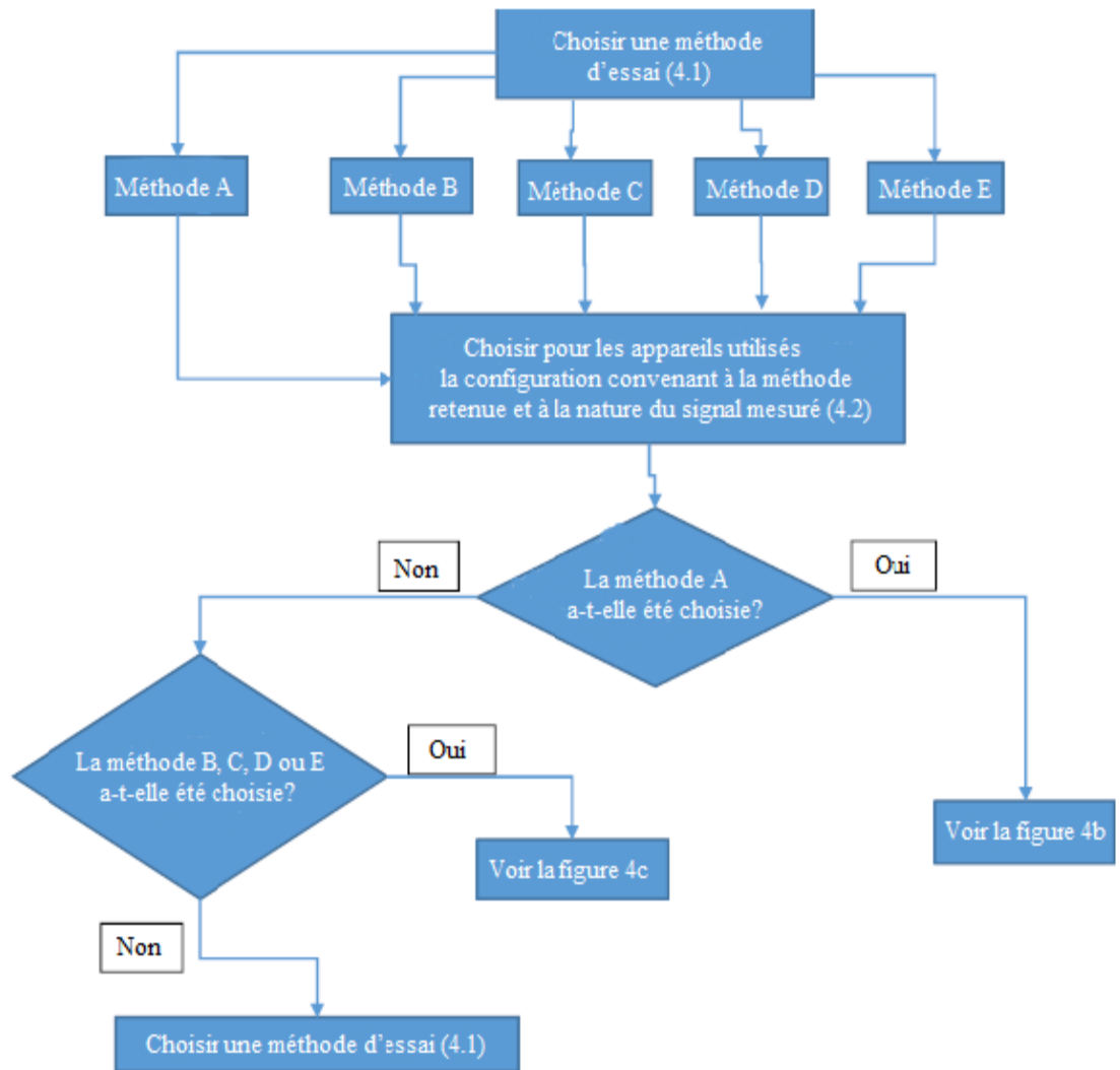
Figure 7a Méthodes d'essai pour la mesure du changement de fréquence
