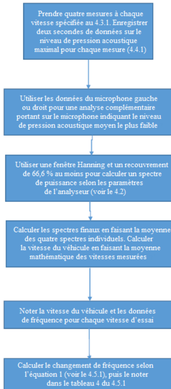
Figure 7b Procédure d'essai pour la mesure du changement de fréquence – méthode A
