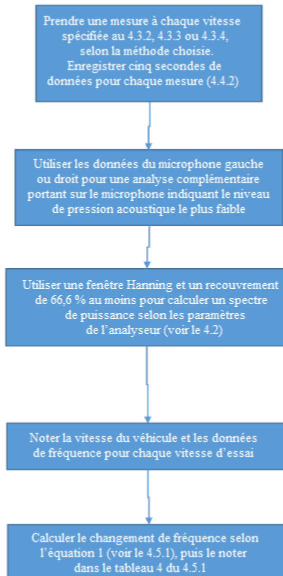
Figure 7c Procédure d'essai pour la mesure du changement de fréquence – méthodes B, C, D et E
