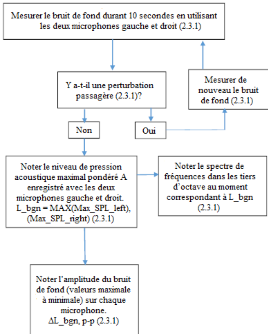
Figure 4 Détermination de l'amplitude du bruit de fond
