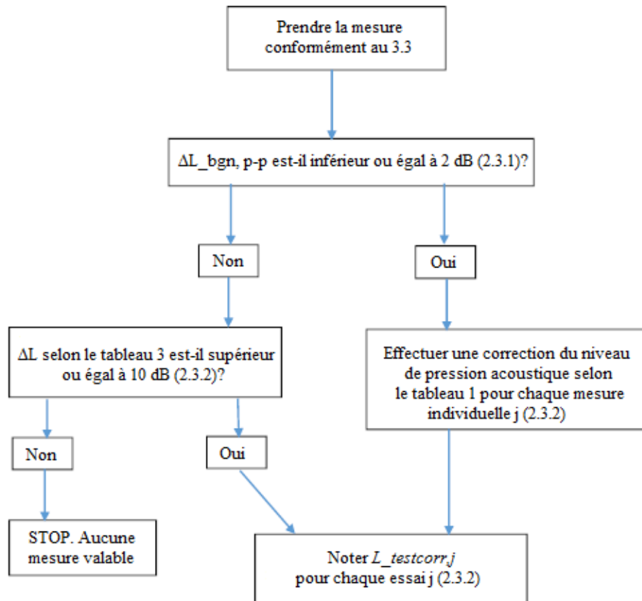
Figure 5 Critères de correction des mesures du niveau de pression acoustique pondéré A du véhicule
